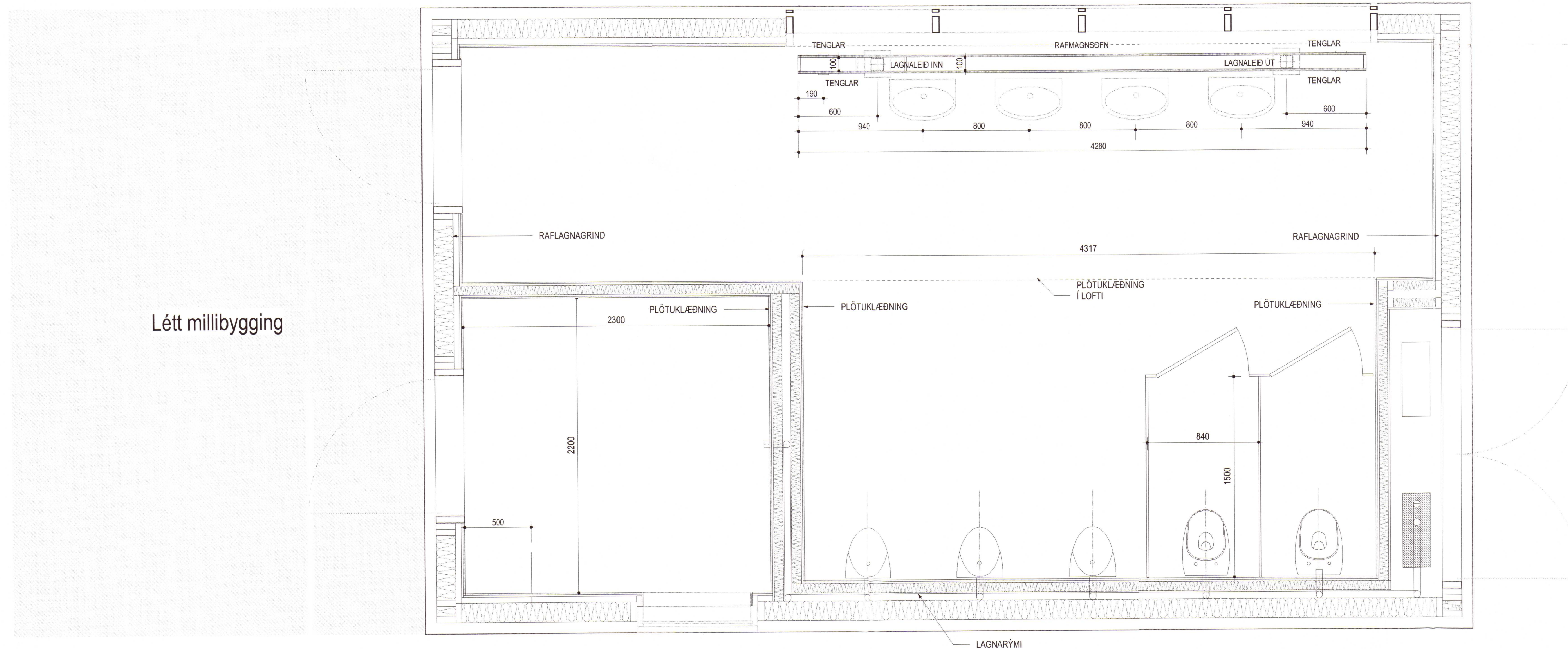
2 GRUNNMYND - SNYRTINGAR KARLA 1:20
