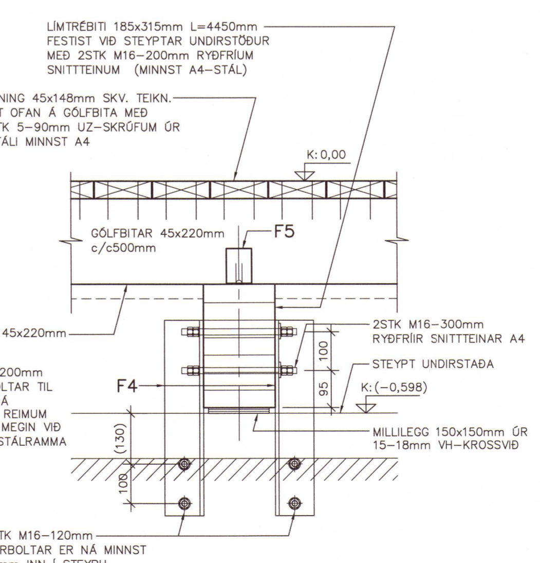
SM8 SÉRMYND 1:10
