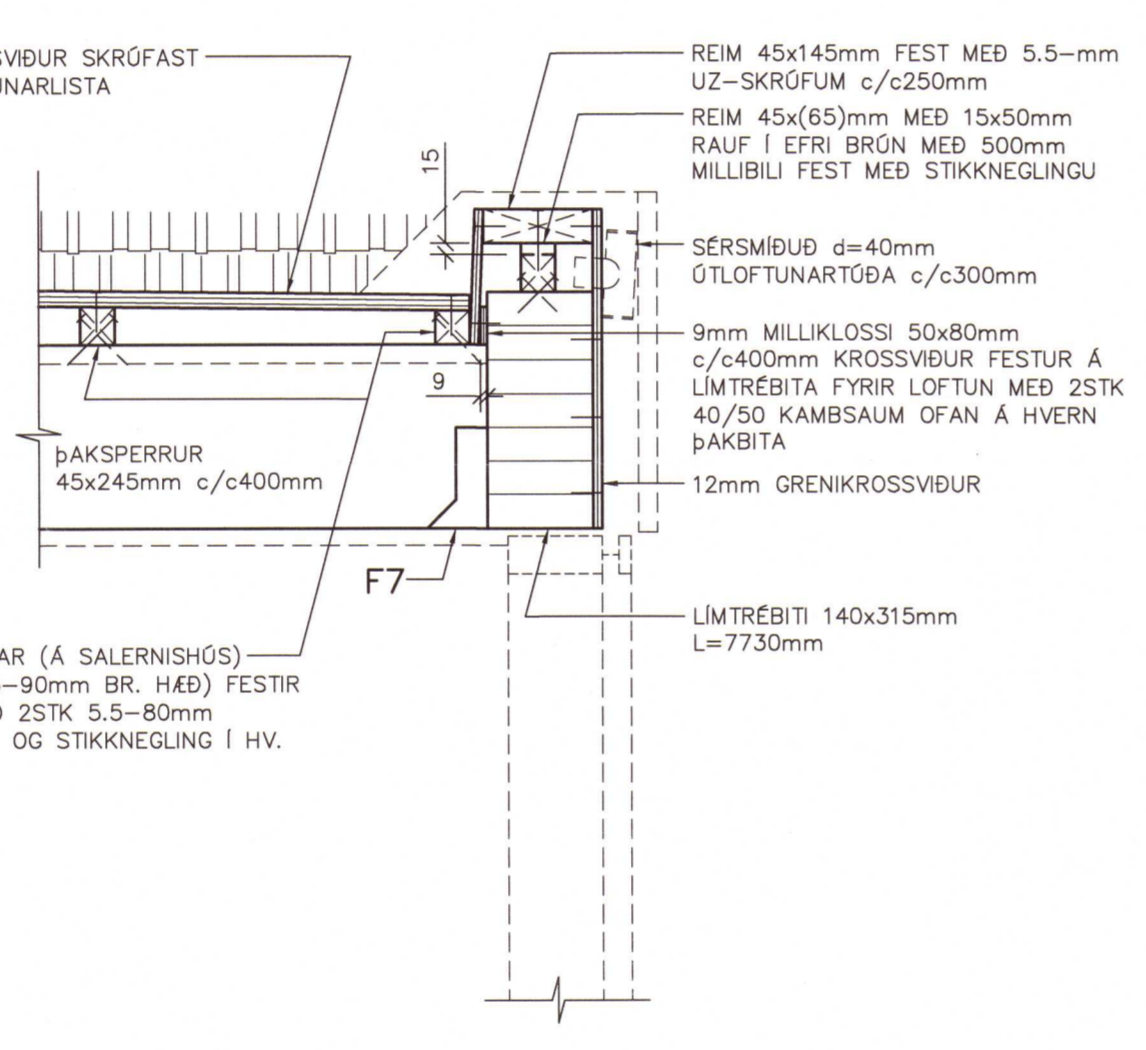
SM6 SÉRMYND 1:10
