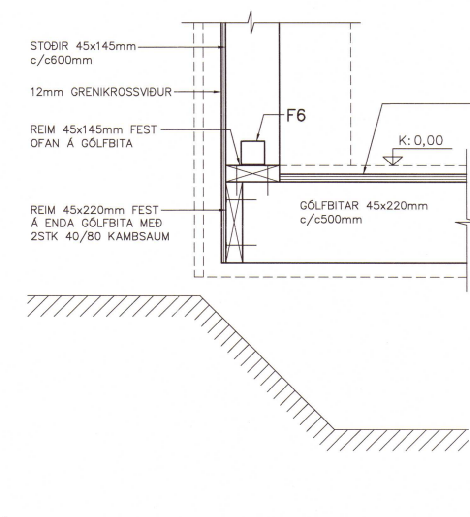
SM7 SÉRMYND 1:10
