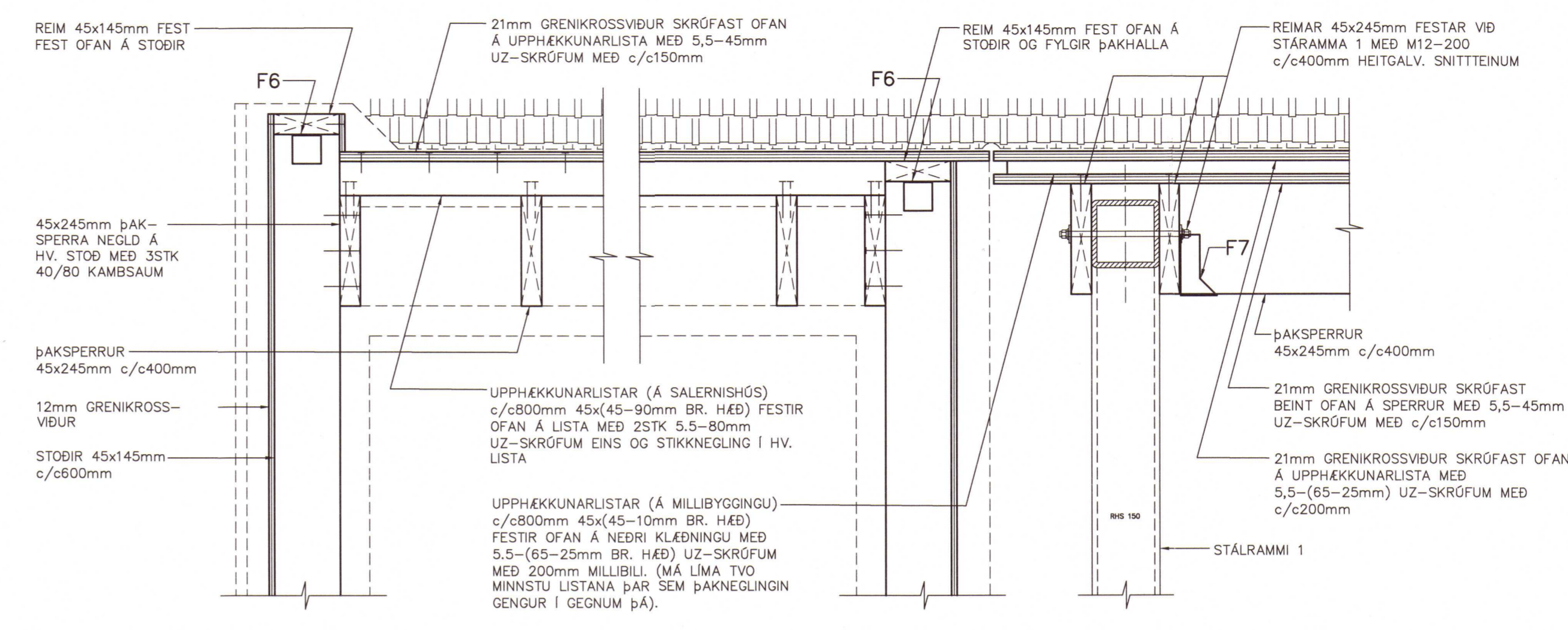
4 SNIÐ 1:10
