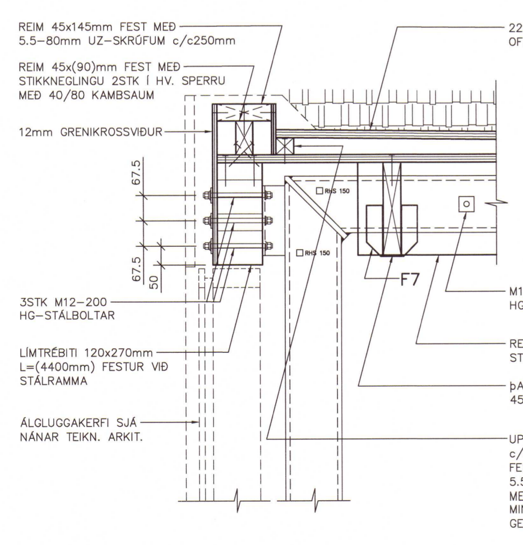
SM5 SÉRMYND 1:10
