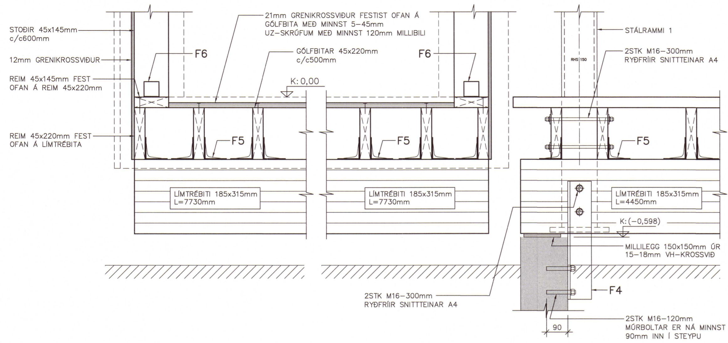
SM1 SÉRMYND 1:10
