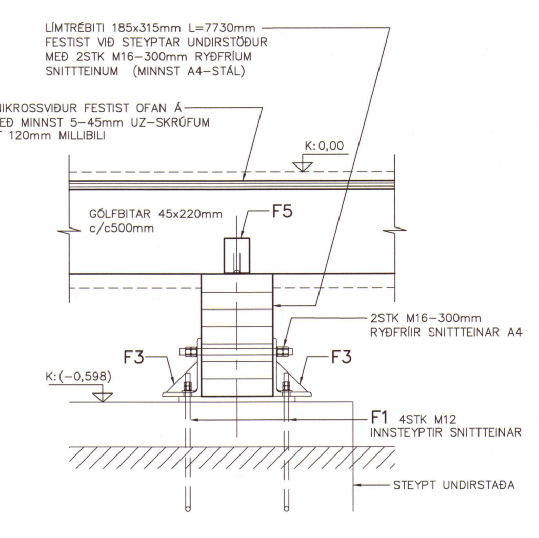
SM8 SÉRMYND 1:10
