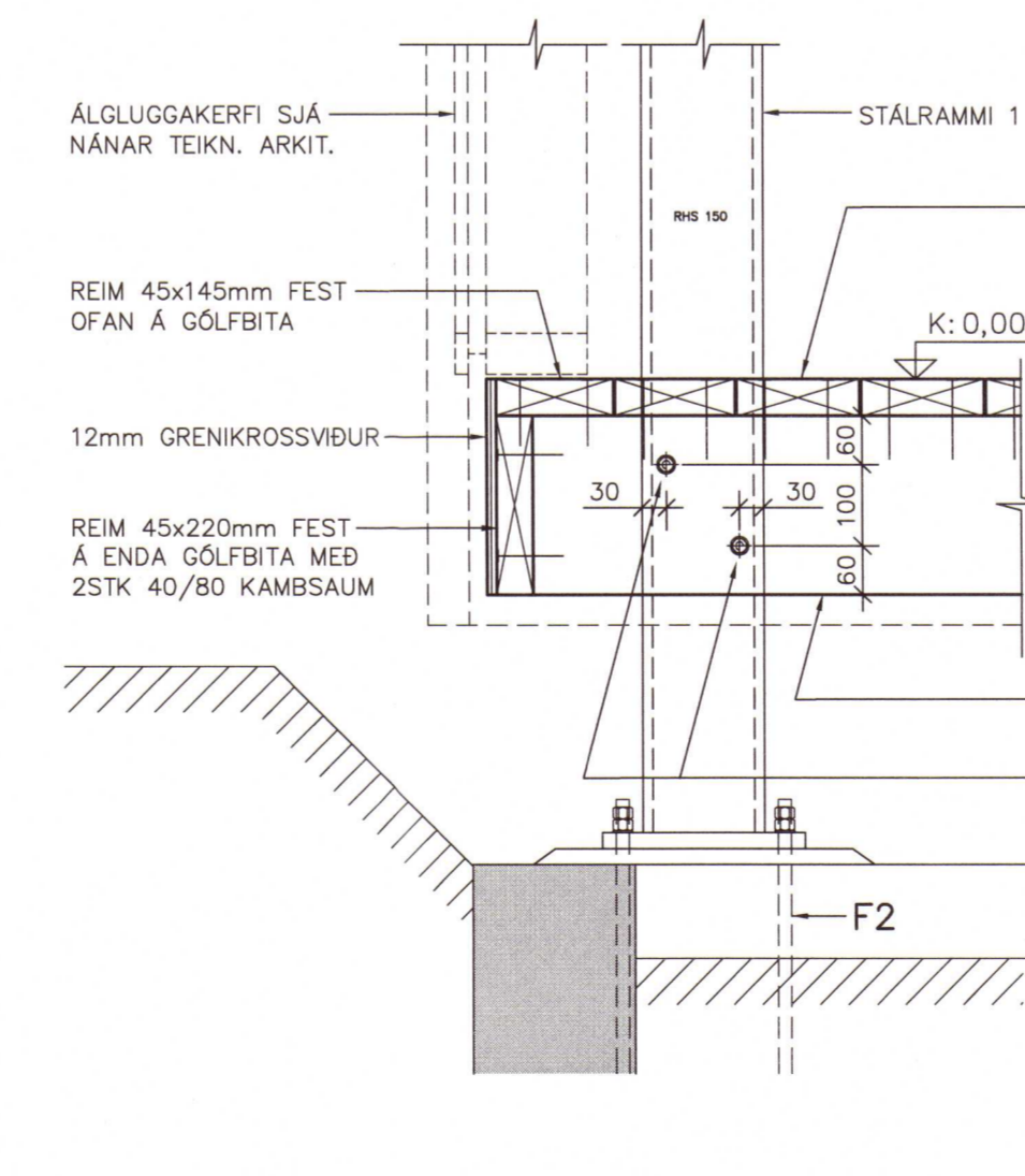
SM7 SÉRMYND 1:10
