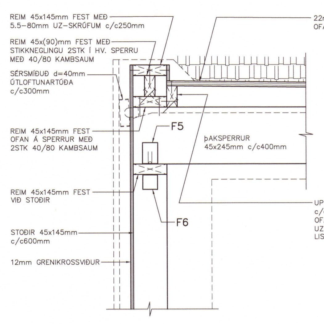
SM5 SÉRMYND 1:10
