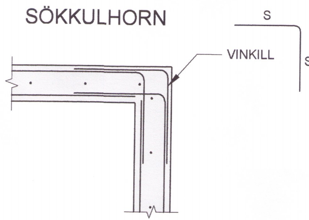
ALMENNT DEILI Mkv. 1:20
