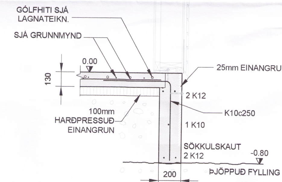
SNIÐ B1 Mkv. 1:20
