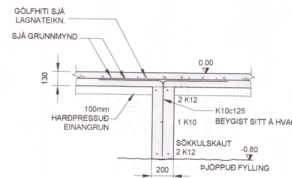
SNIÐ B2 Mkv. 1:20
