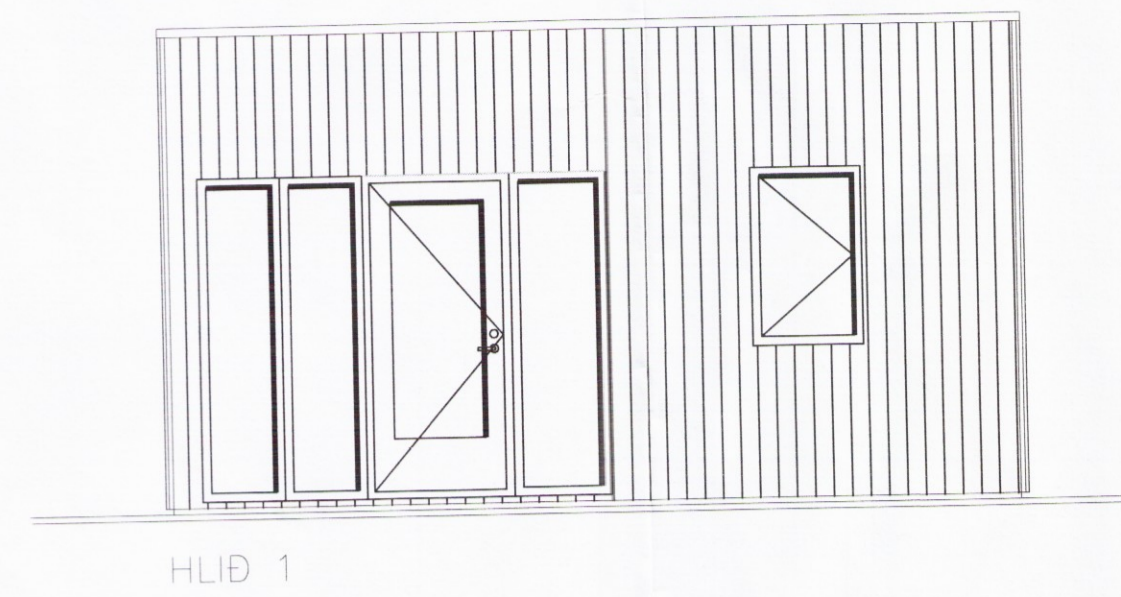
HLIÐ 1
