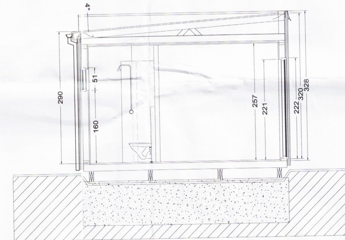
SNIÐ A-A
