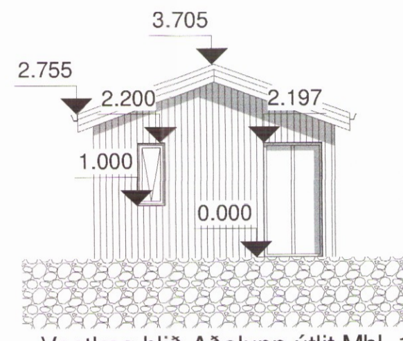
Vestlæg hlið Aðalupp útlit Mhl. 1 1 : 100
