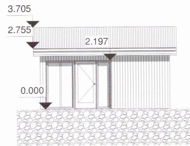
Suðlæg hlið Aðalupp útlit Mhl. 1 1 : 100
