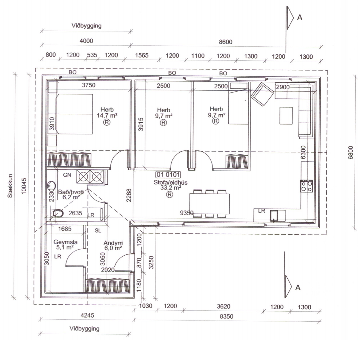
Grunnmynd 1:100
