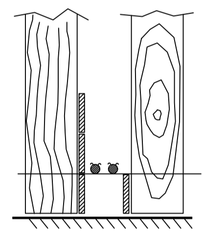
SNID A - A Í SÖKKULVEGG SÝND ERU 2 NEDSTU STEYPU- STYRKJARJÄRN Í STEYPUÖTI OFAN Á NEDSTU MOTAVÍRUM
