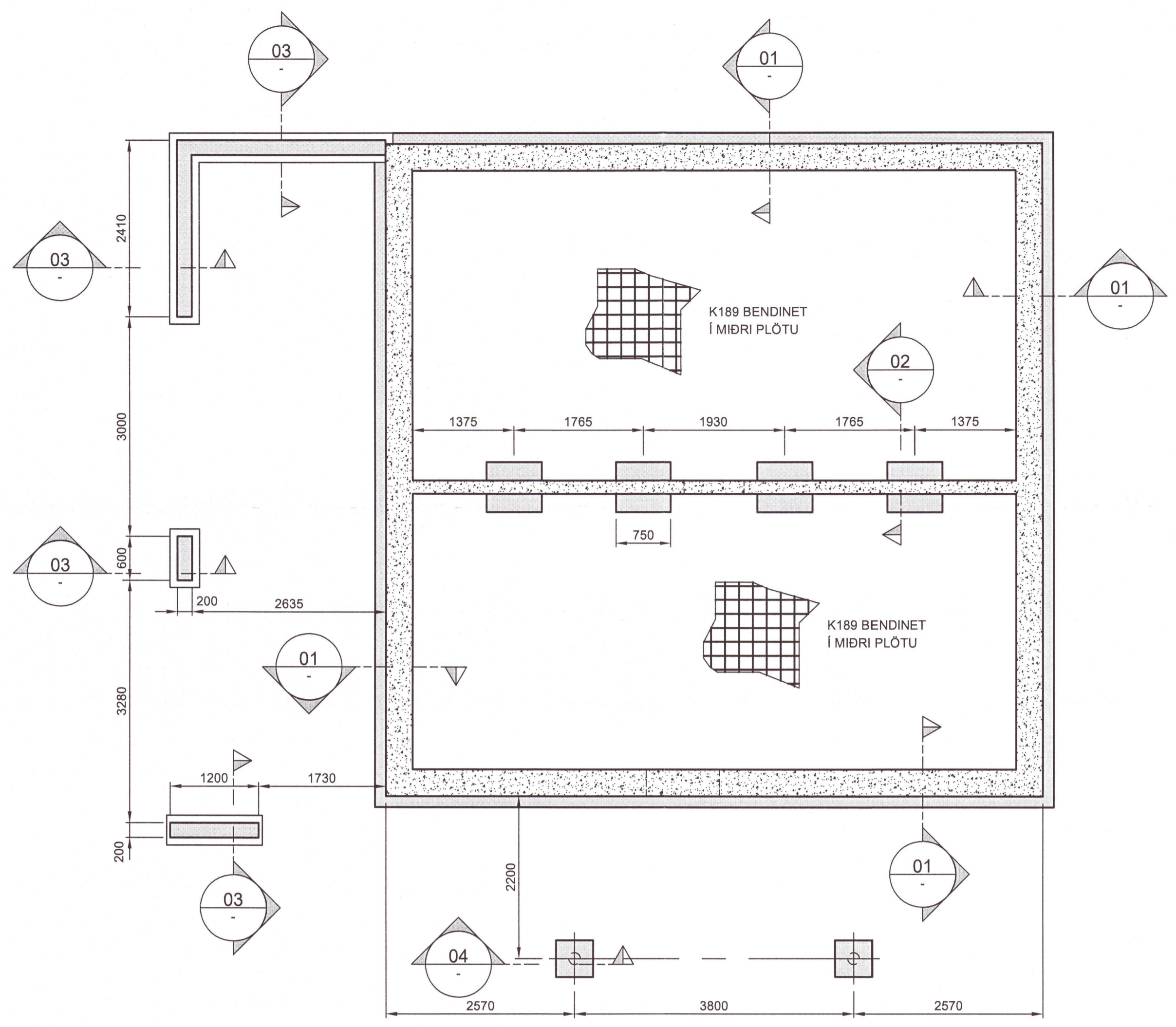
GRUNNMYND UNDIRSTÖÐUR MKV. 1:50
