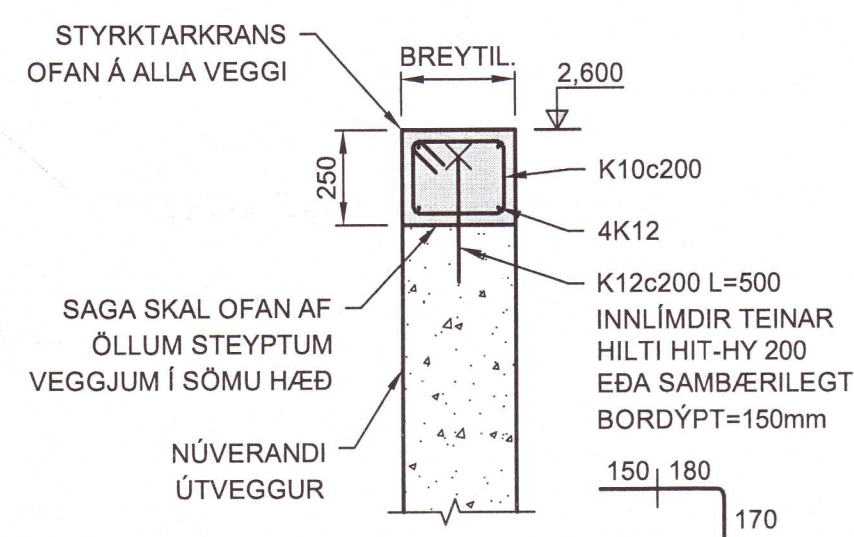
15 SNID - 15* ER SAMSKONAR 1:20
