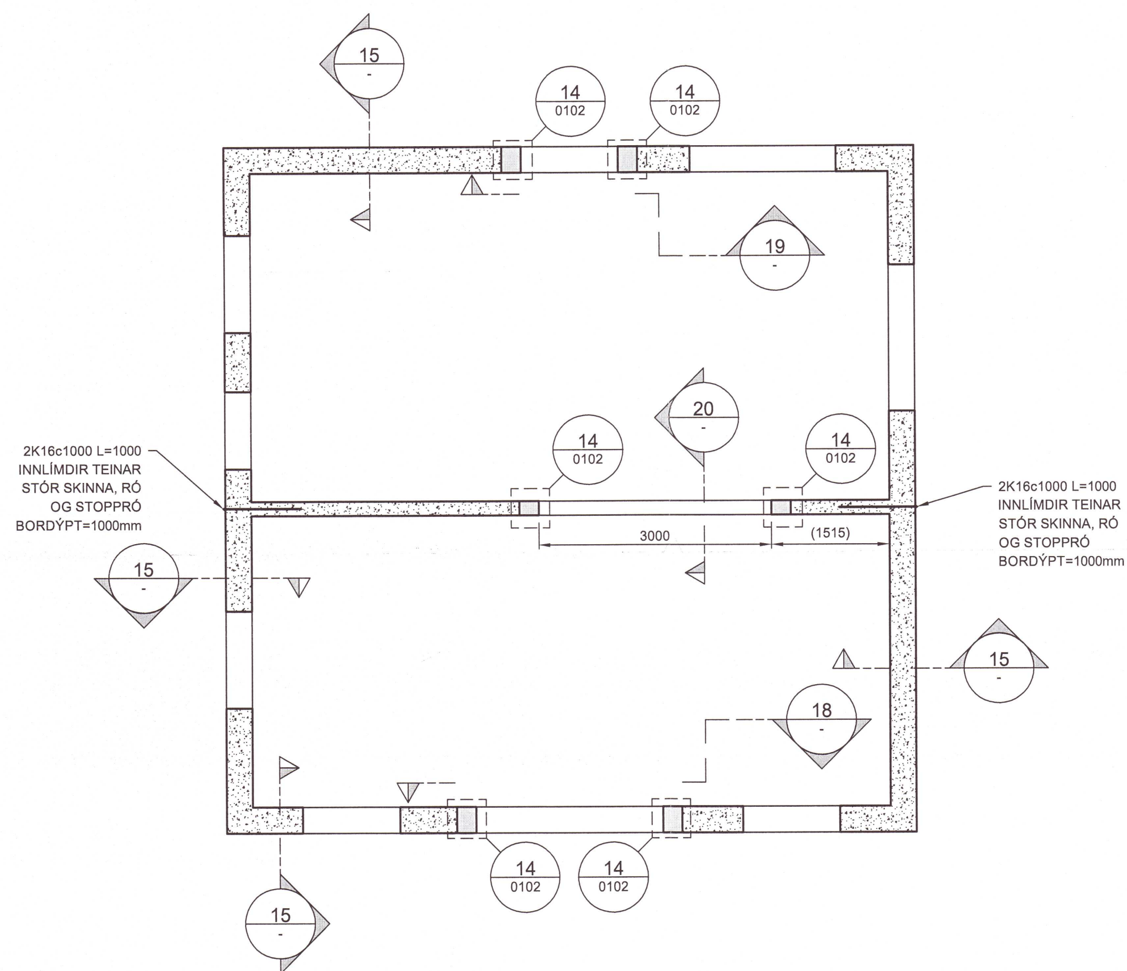
GRUNNMYND, 1.HÆÐ MKV. 1:50
