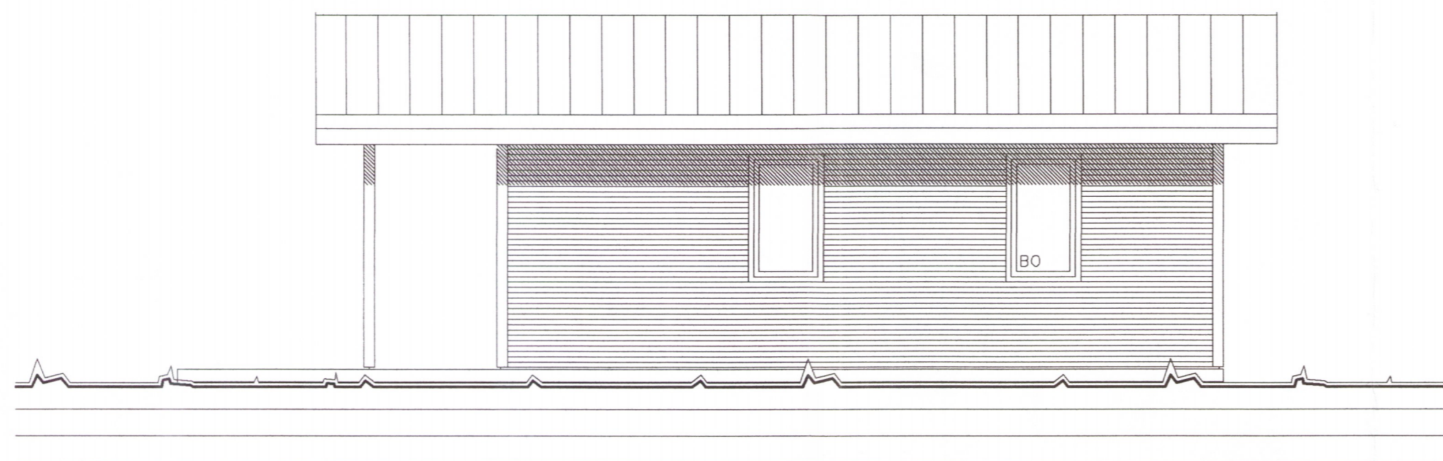
NORÐ - AUSTUR
