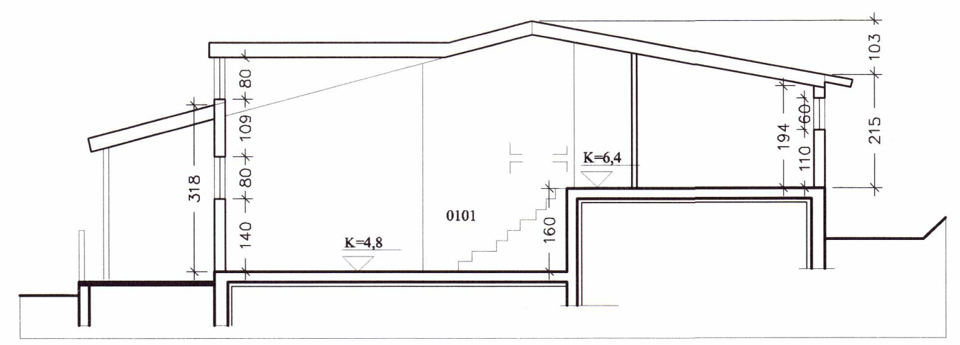
SNEIÐING a-a 1:100
