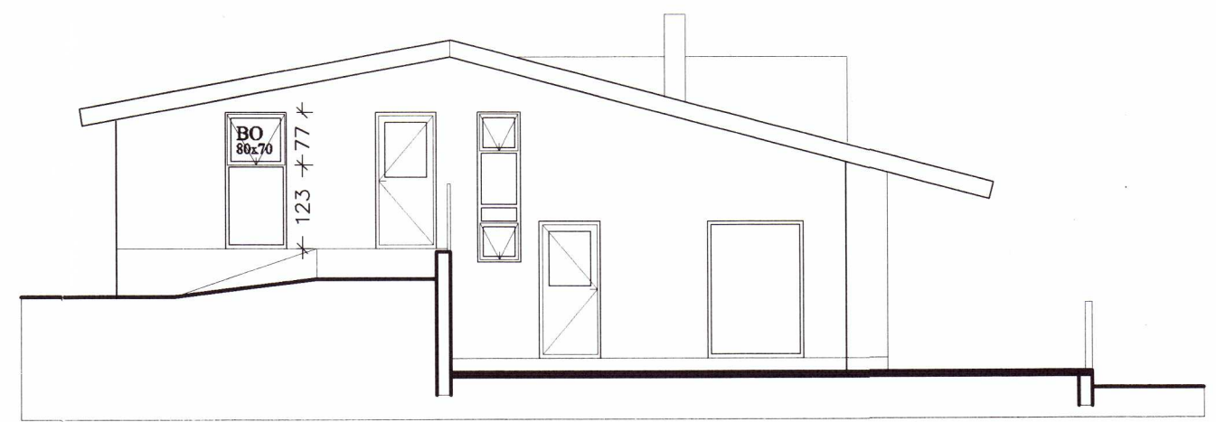
ÚTLIT NORÐUR 1:100
