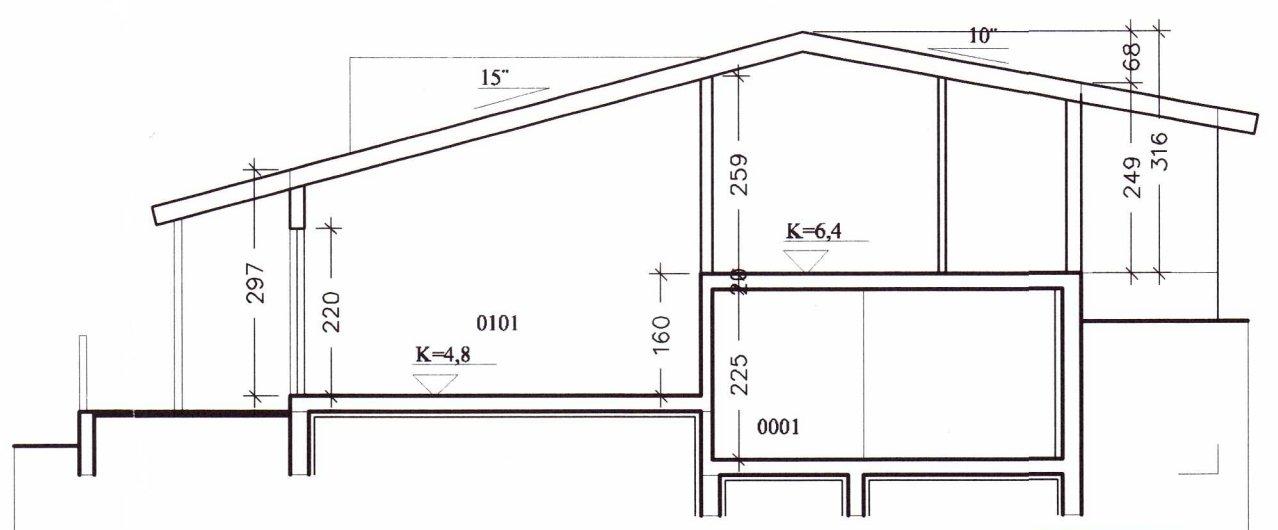
SNEIÐING b-b 1:100
