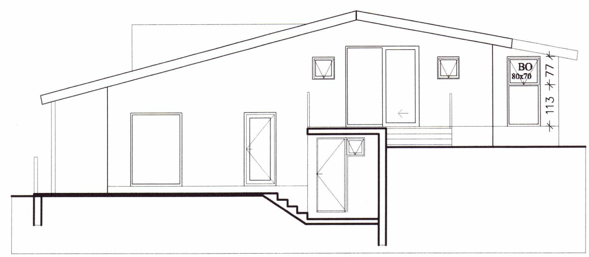
ÚTLIT SUÐUR 1:100
