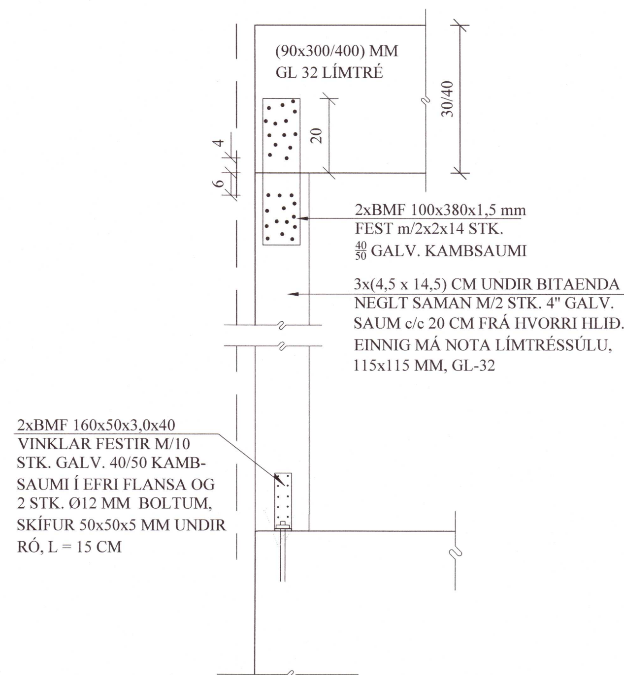
SM1 1-03 SÉRMYND. 1:10 FESTINGAR LÍMTRÉBITA VIÐ ÚTVEGGI
