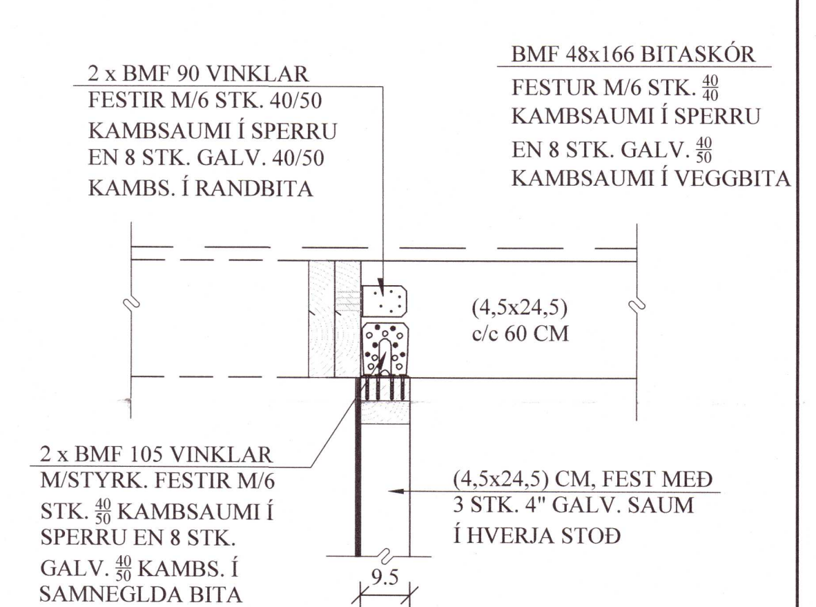
E3 1-03 SNIÐ. 1:10
