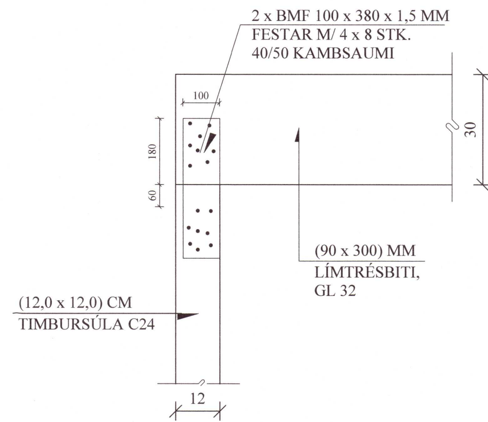
S1 1-03 SÉRMYND. 1:10 TIMBURSÚLUR ÚTI
