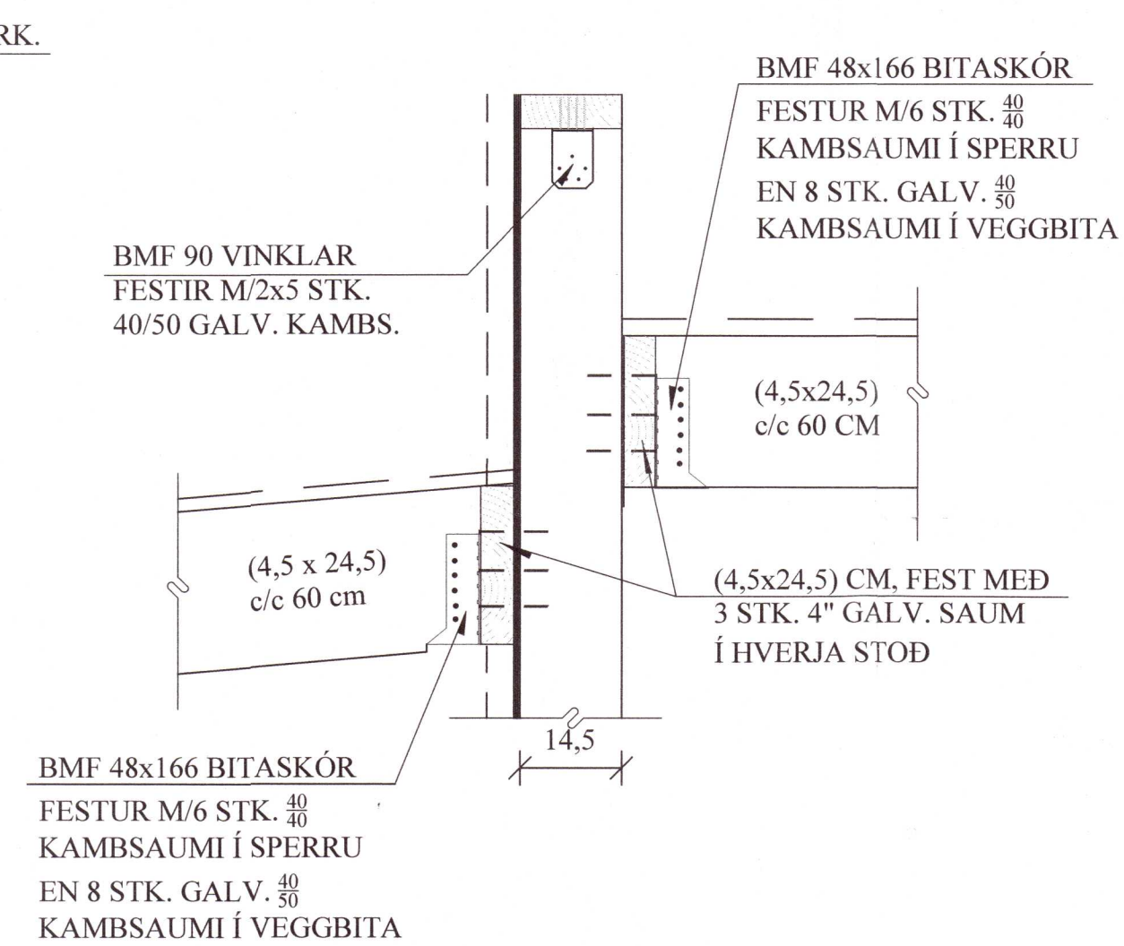
D3 1-03 SNIÐ. 1:10
