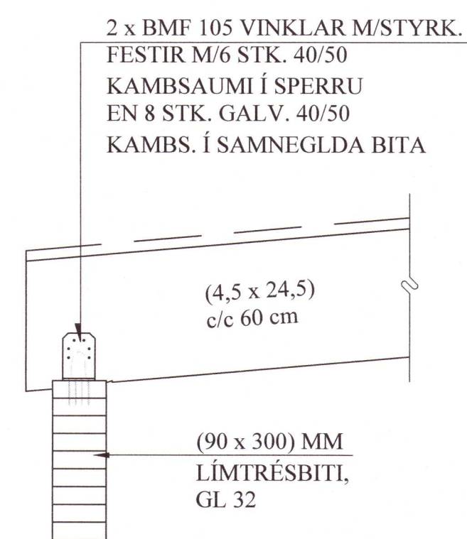
C3 1-03 SNIÐ. 1:10 Í SNIÐI C3' ER LÍM- TRÉSBITI (90x400) MM
