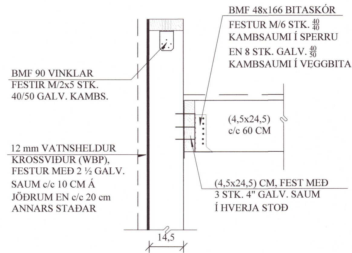
C3 1-03 SNIÐ. 1:10 Í SNIÐI C3' ER LÍM- TRÉSBITI (90x400) MM
