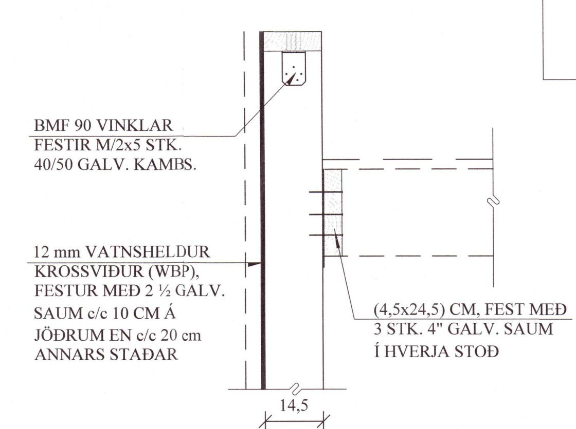
D3 1-03 SNIÐ. 1:10
