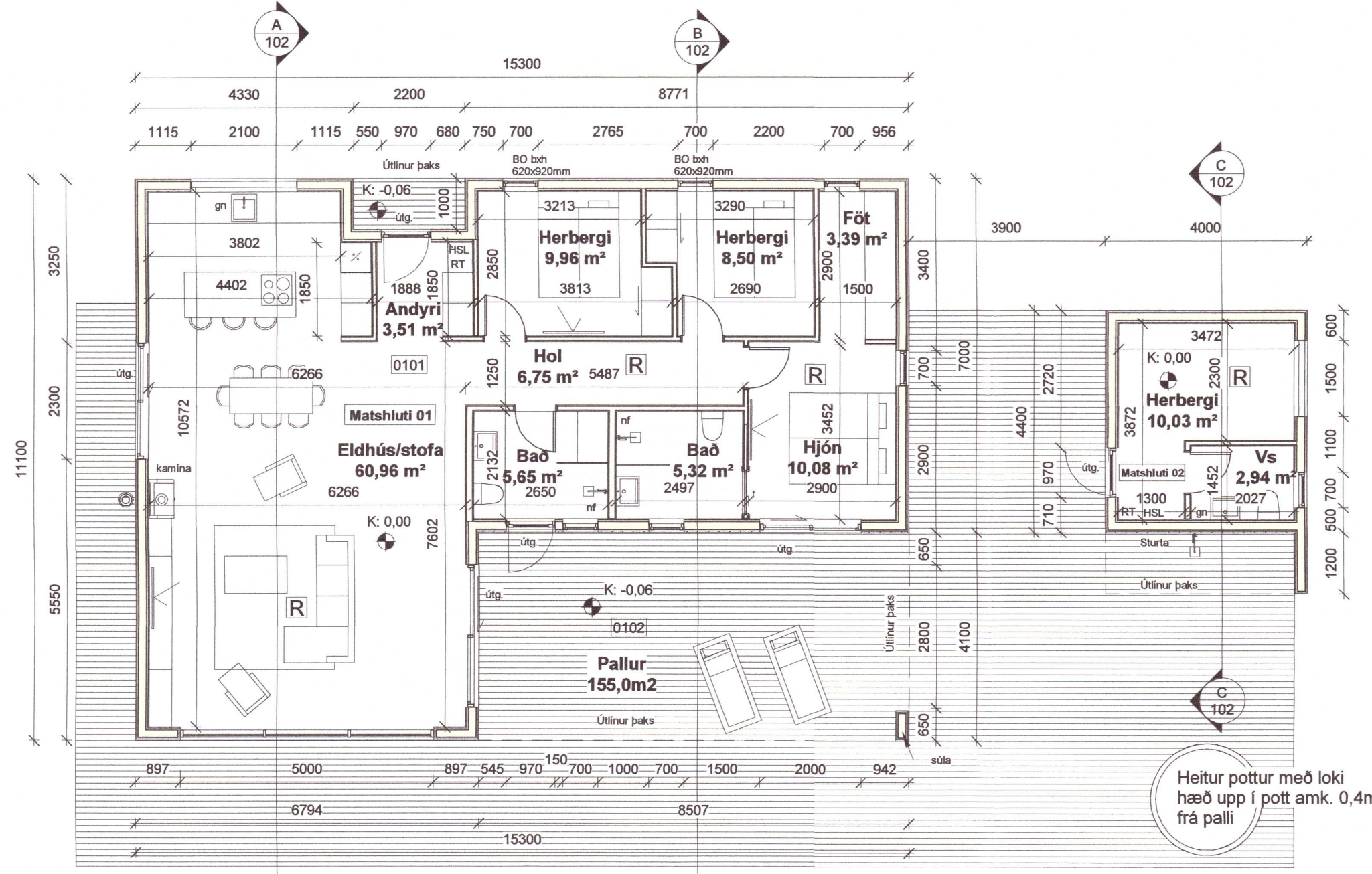
1 1. Hæð 1 : 100
