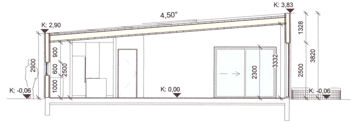
A Snið A 1 : 100
