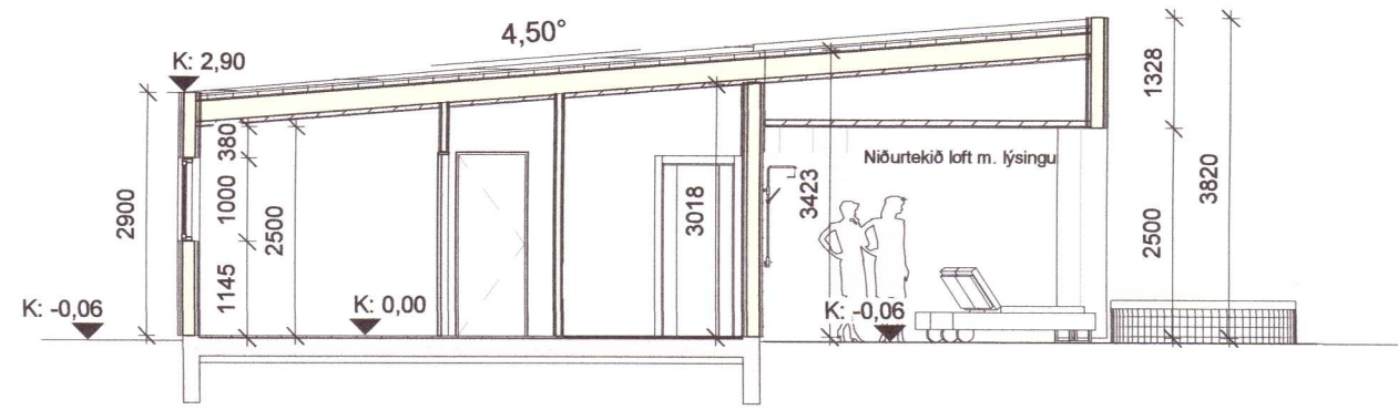
B Snið B 1 : 100
