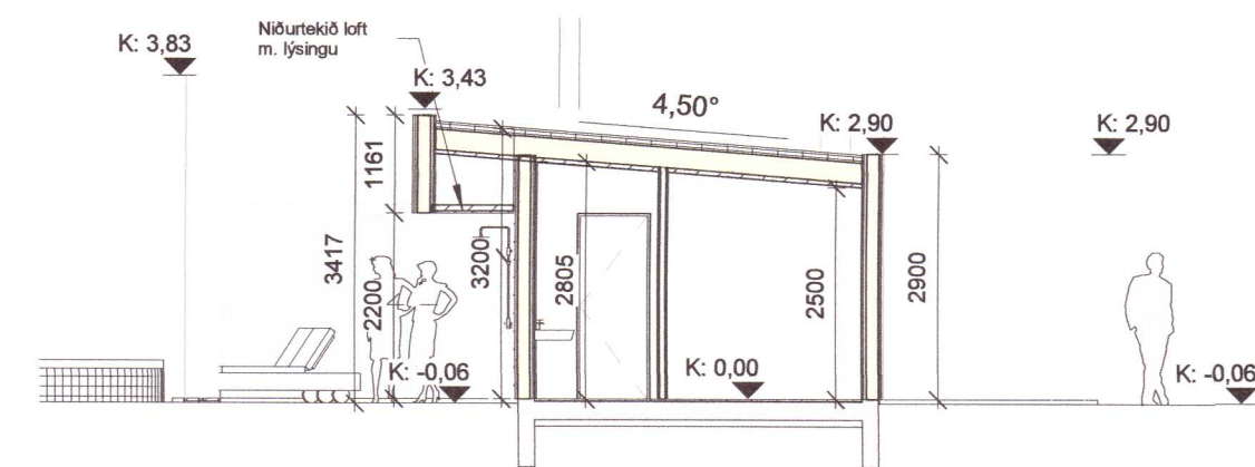
C Snið C 1 : 100
