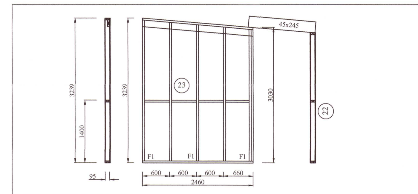
Burðarveggir innanhúss MKV. 1:50
