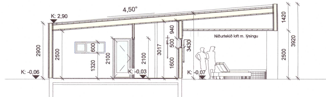
B Snið B 1 : 100
