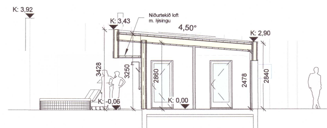
C Snið C 1 : 100
