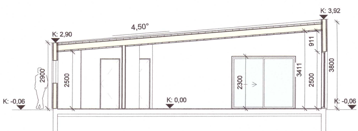
A Snið A 1 : 100
