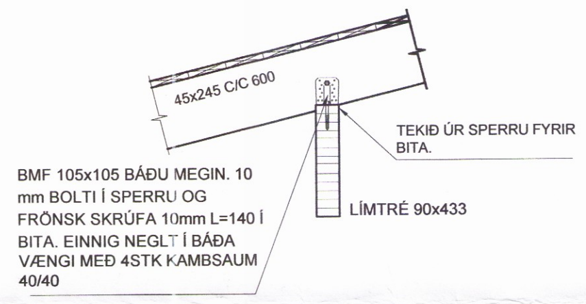
K SNÍÐ B4 M. 1: 20
