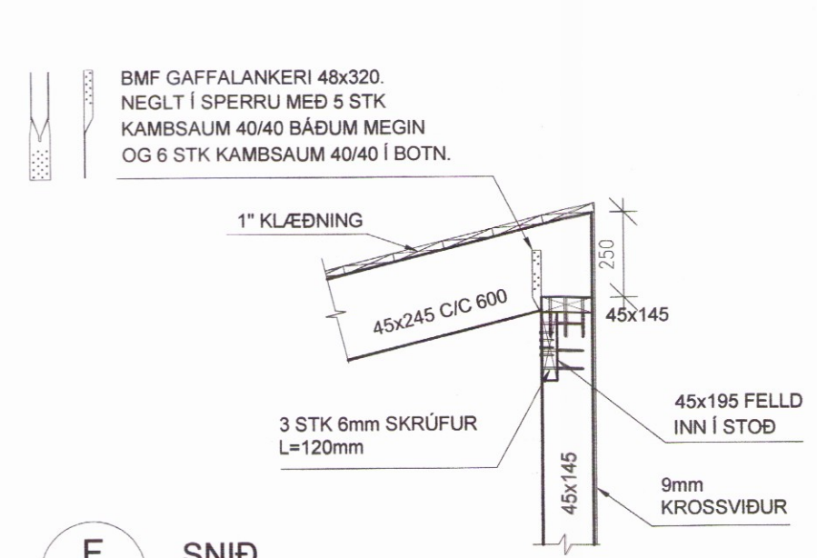
F SNÍÐ B4 M. 1: 20
