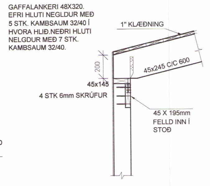
G SNÍÐ B4 M. 1: 20
