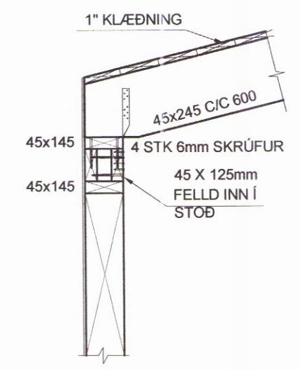
H SNÍÐ B4 M. 1: 20
