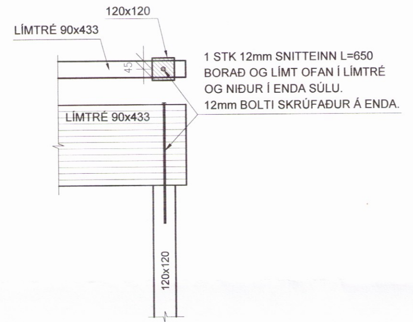
I SNÍÐ B4 M. 1: 20
