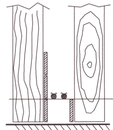
SNID A - A Í SÖKKULVEGG SÝND ERU 2 NEDSTU STEYPU- STYRKJARJÁRN Í STEYPUMÓTI OFAN Á NEDSTU MÓTAVÍRUM
