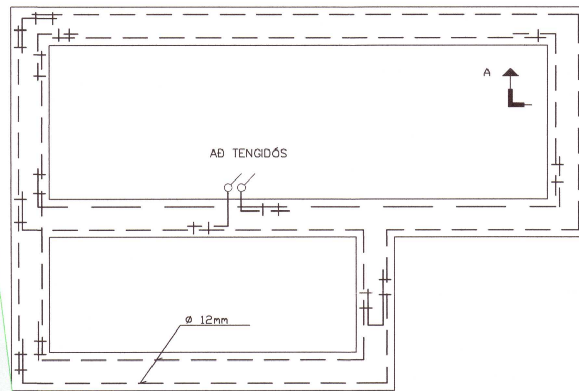
GRUNNMYND SÖKKULVEGGJA
