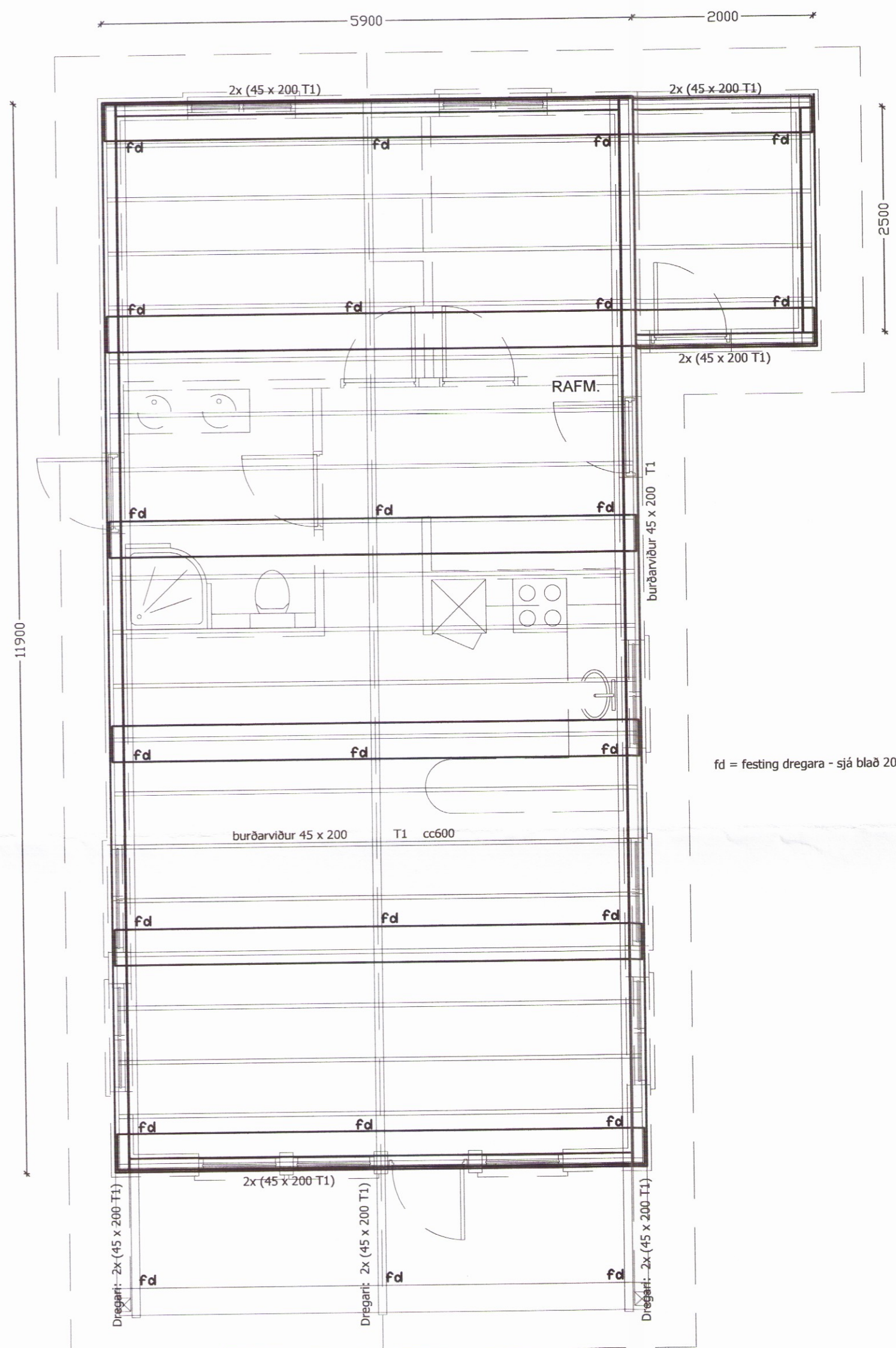
Grunnmynd gólfbita 1:50
