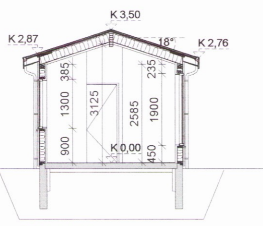
SNID A-A 1:100
