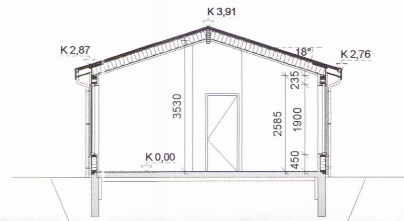
SNID A-A 1:100
