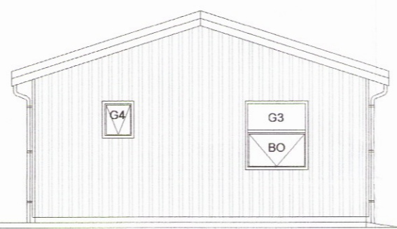
ÚTLIT VESTUR 1:100
