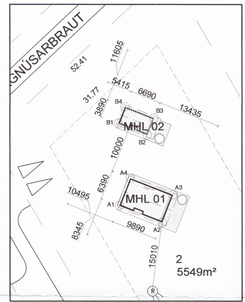
AFSTÖÐUMYND 1:500
