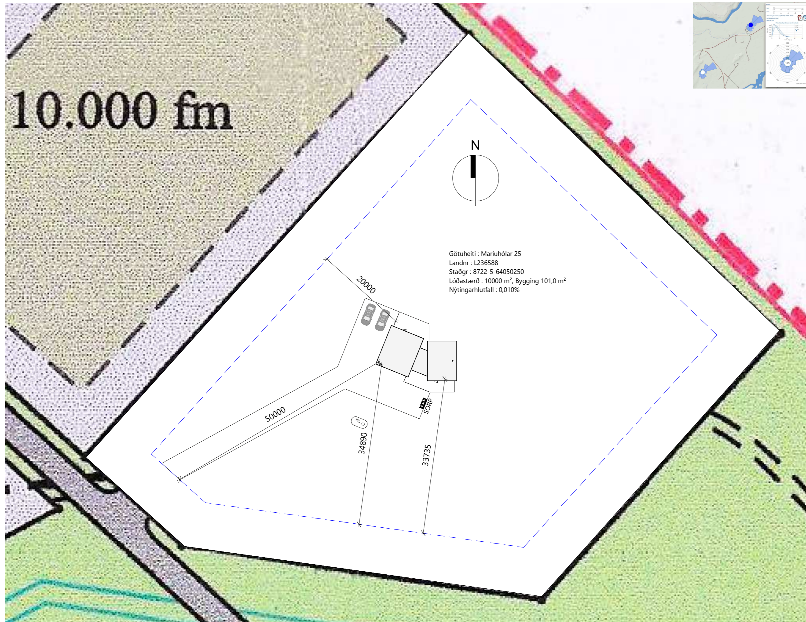
Afstöðumynd 1 : 500
