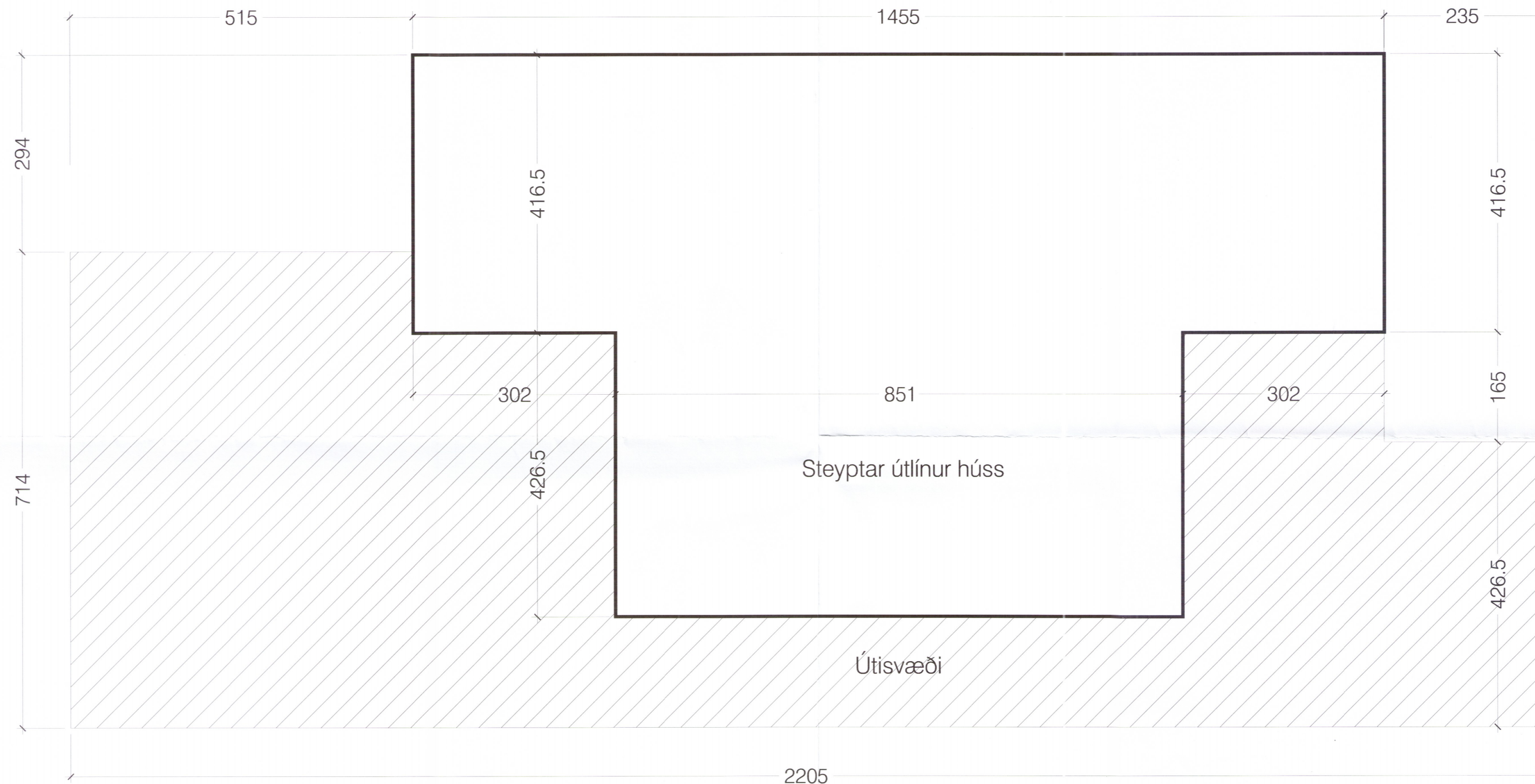
Grunnmynd - mkv. 1:50
