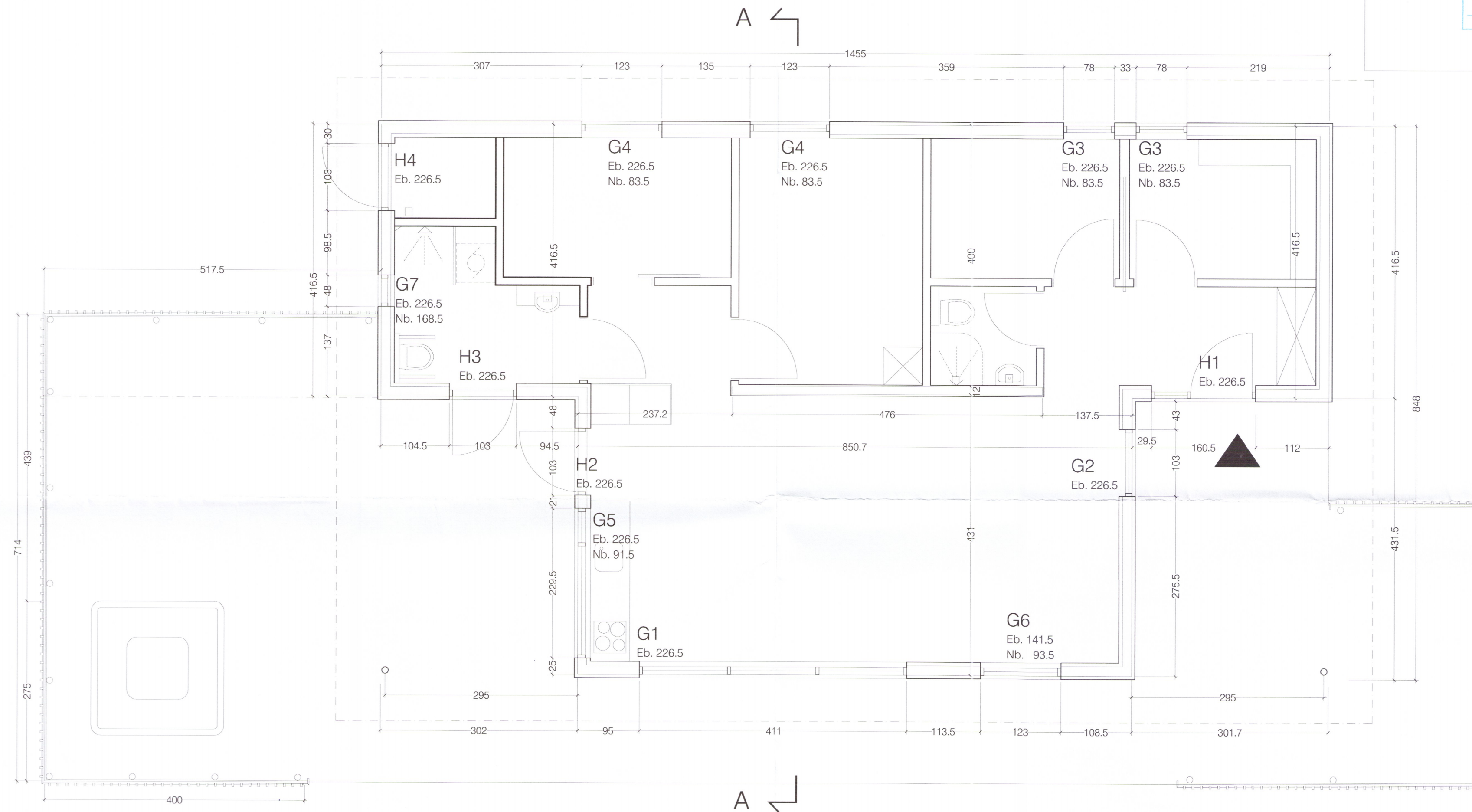
Grunnmynd - mkv. 1:50
