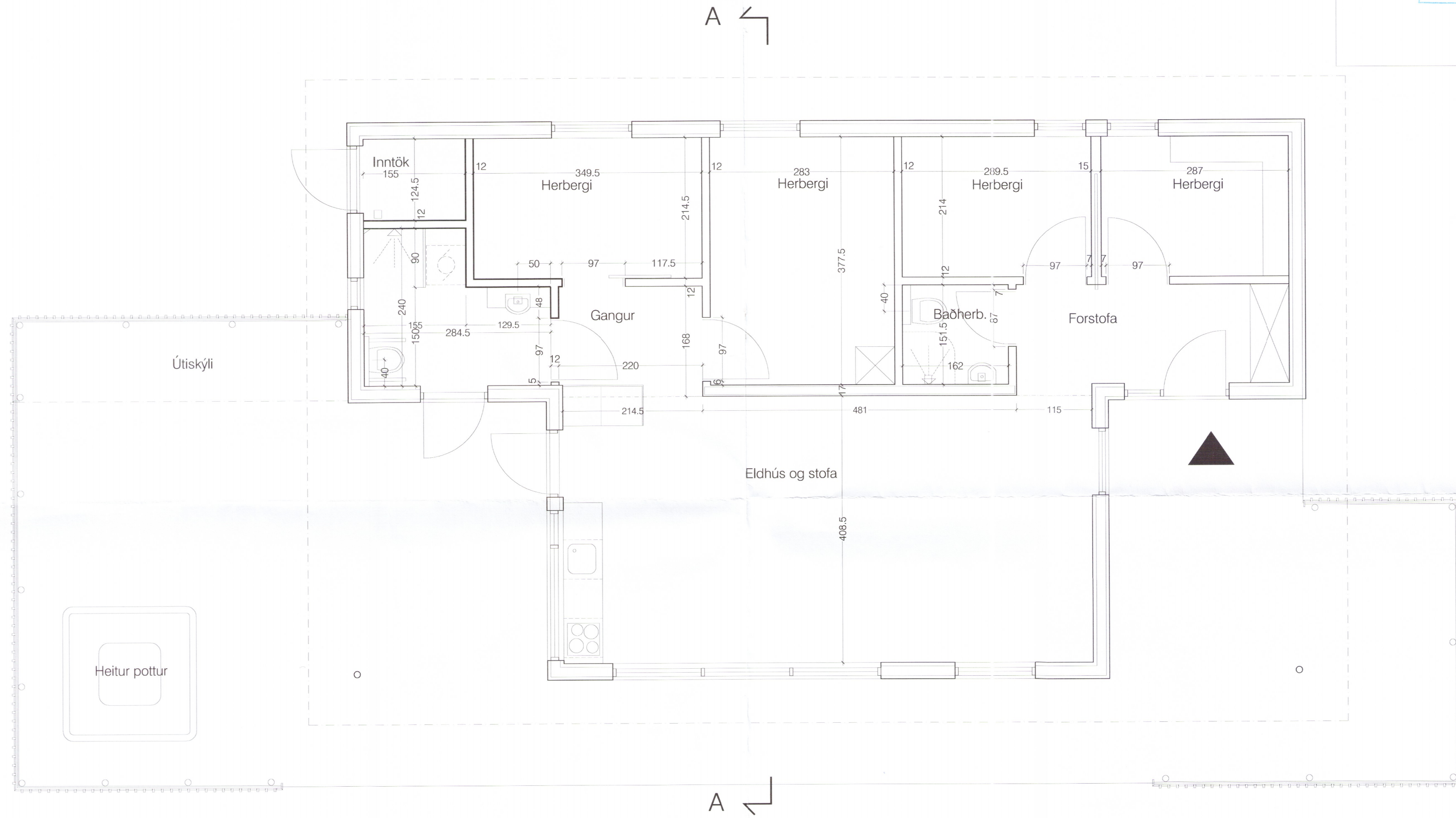
Grunnmynd - mkv. 1:50
