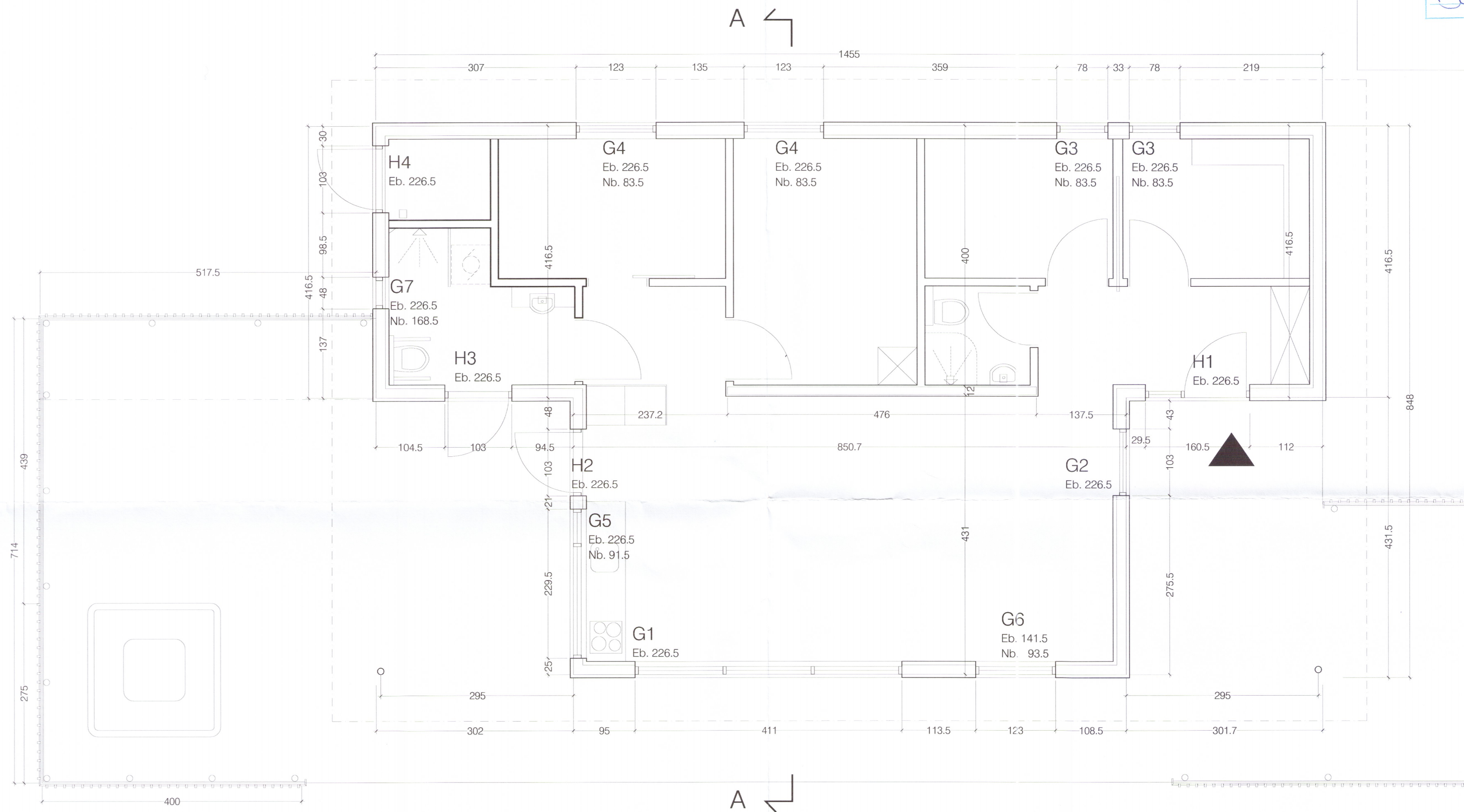
Grunnmynd - mkv. 1:50
