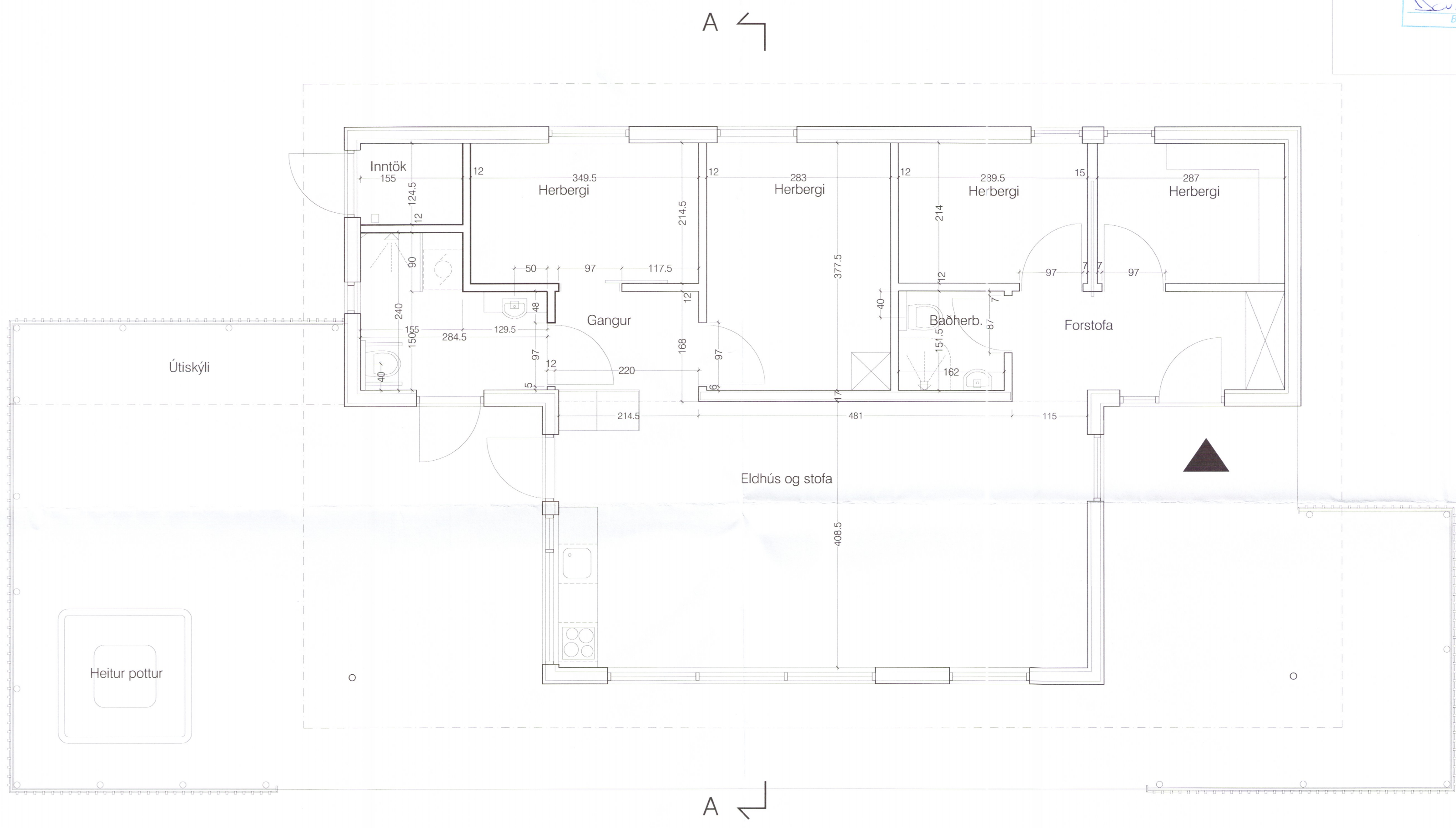
Grunnmynd - mkv. 1:50
