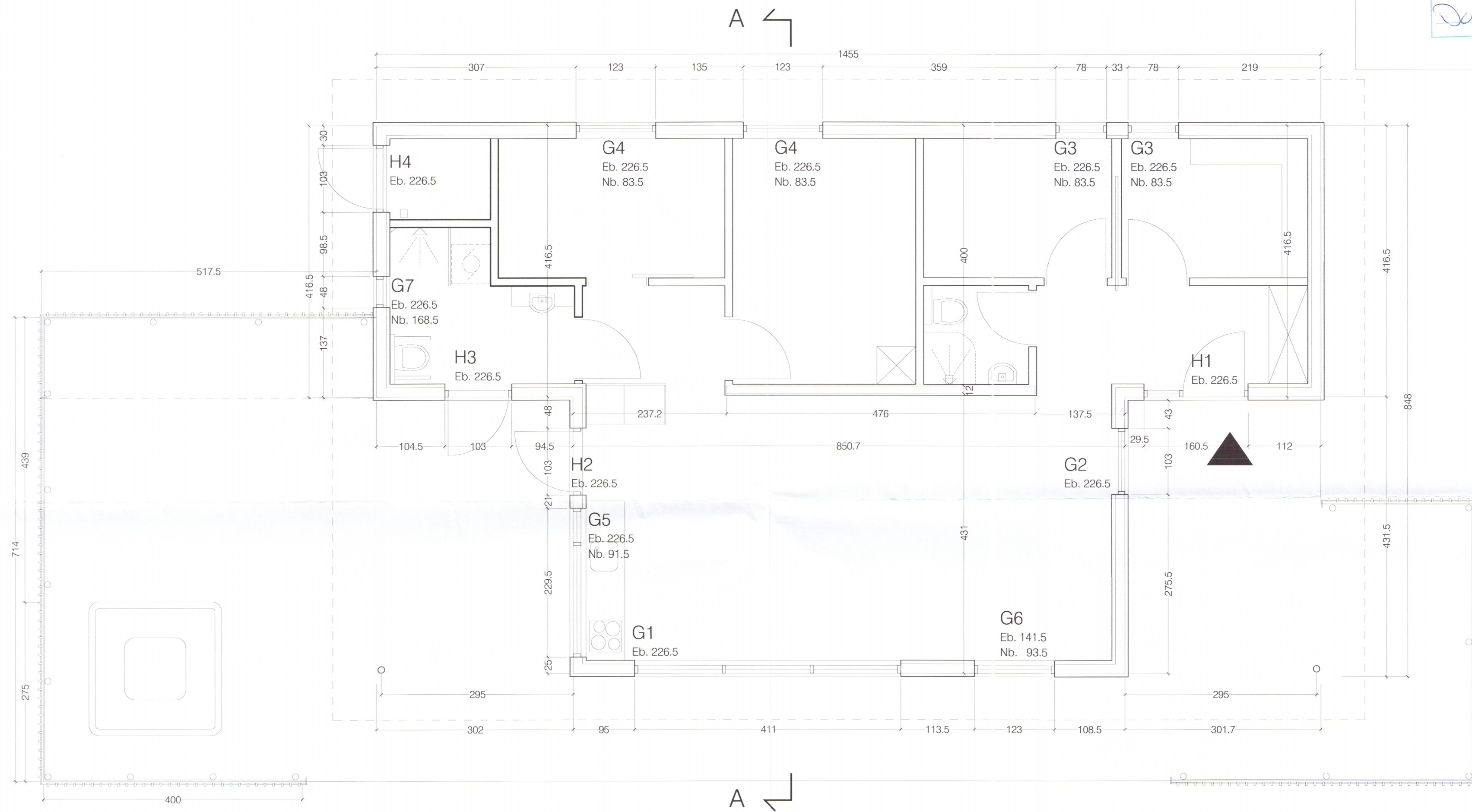
Grunnmynd - mkv. 1:50
