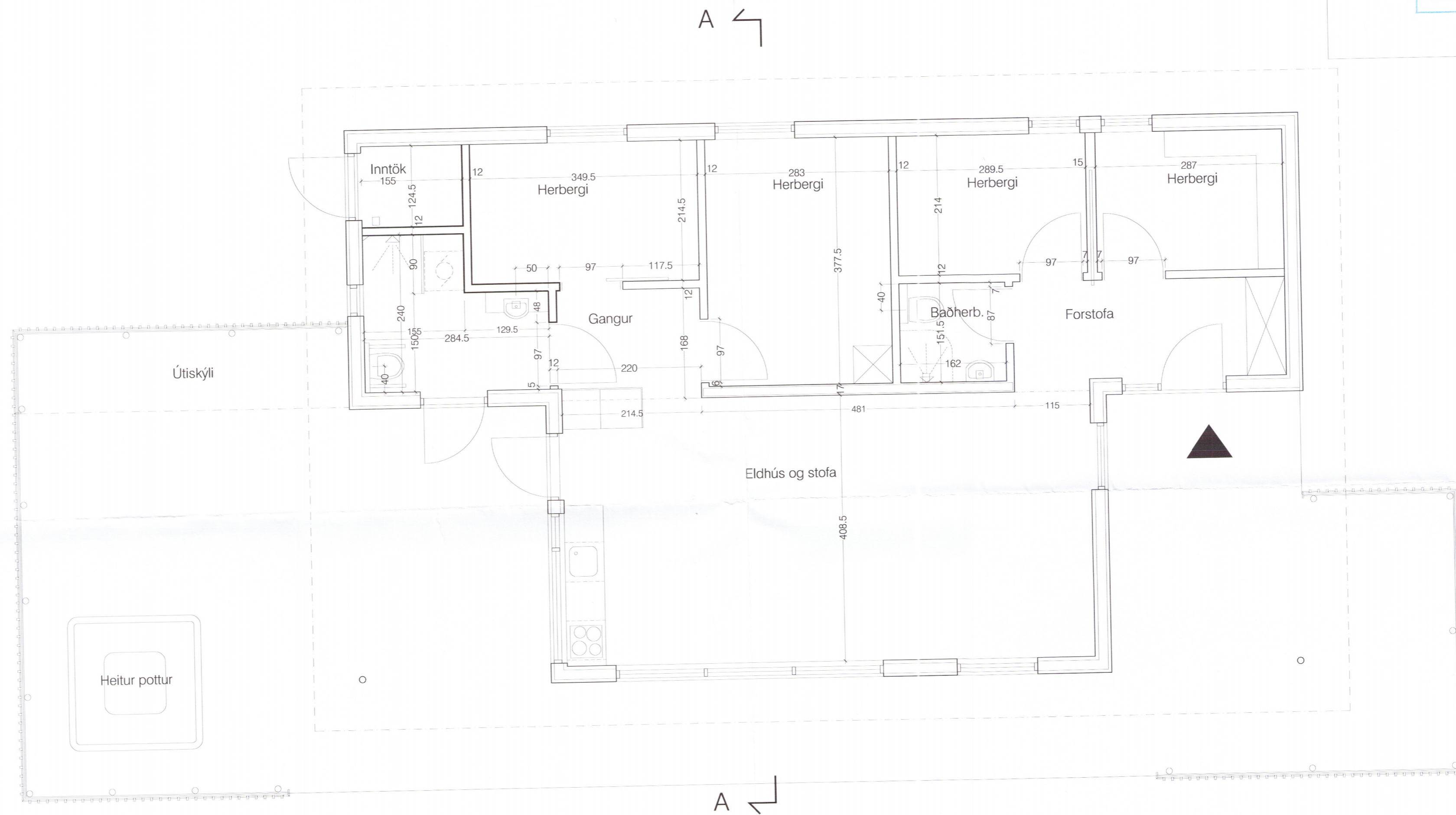
Grunnmynd - mkv. 1:50
