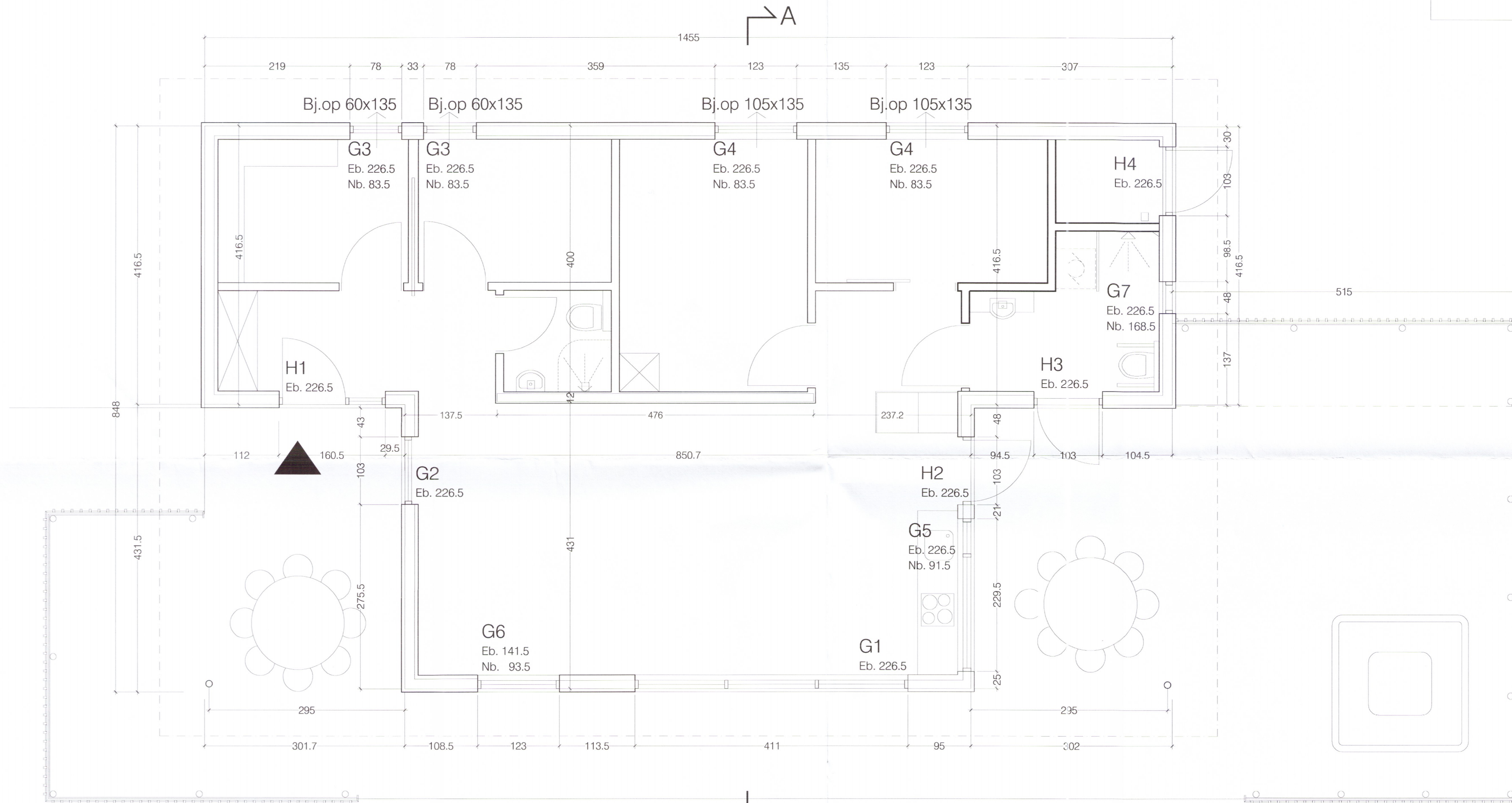
Grunnmynd - mkv. 1:50
