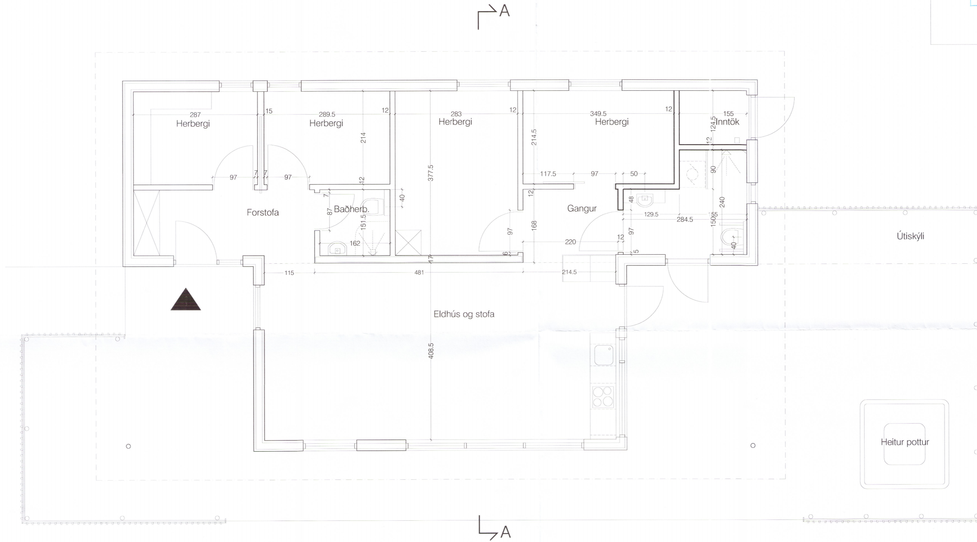
Grunnmynd - mkv. 1:50
