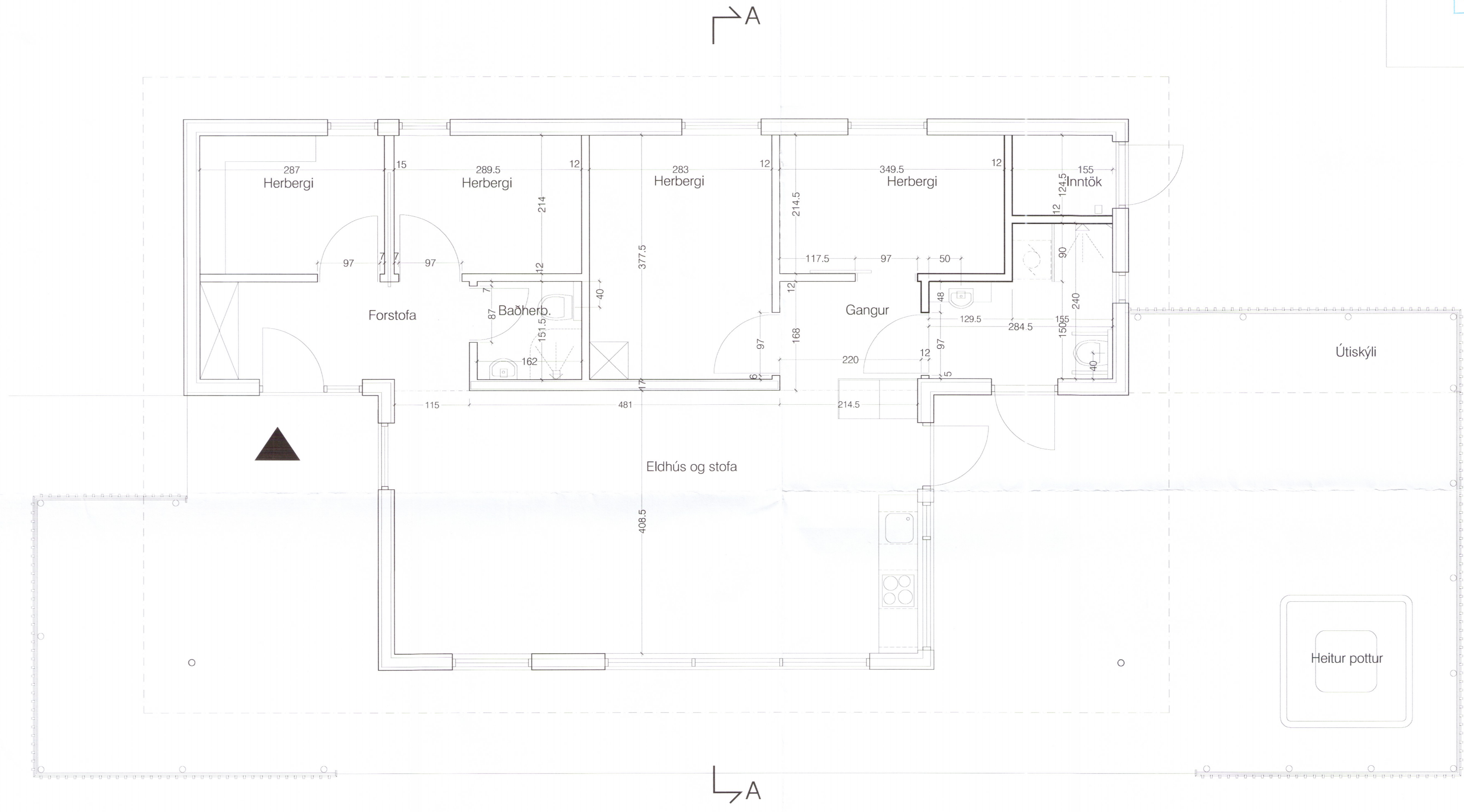
Grunnmynd - mkv. 1:50
