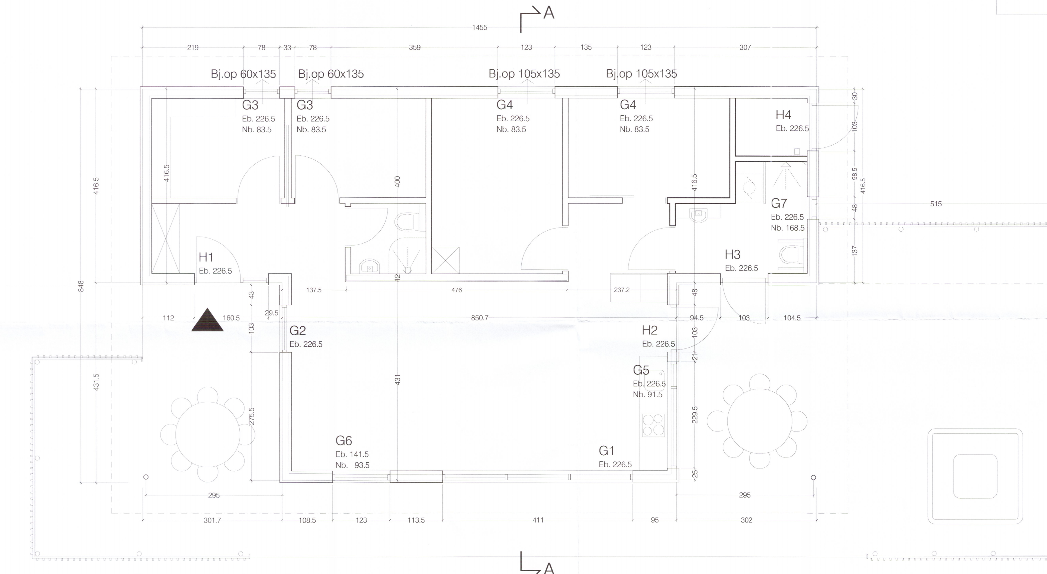
Grunnmynd - mkv. 1:50
