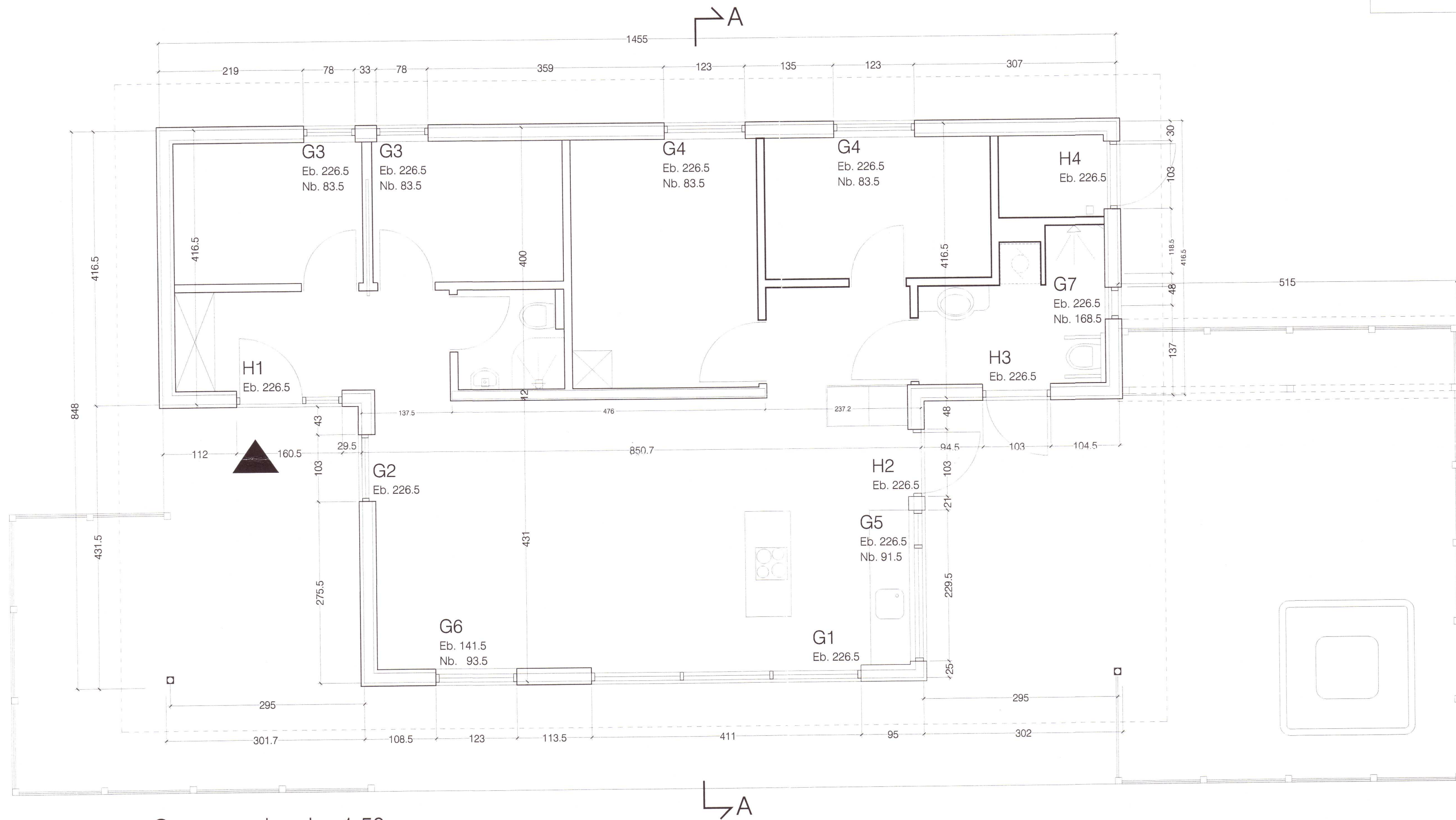
Grunnmynd - mkv. 1:50
