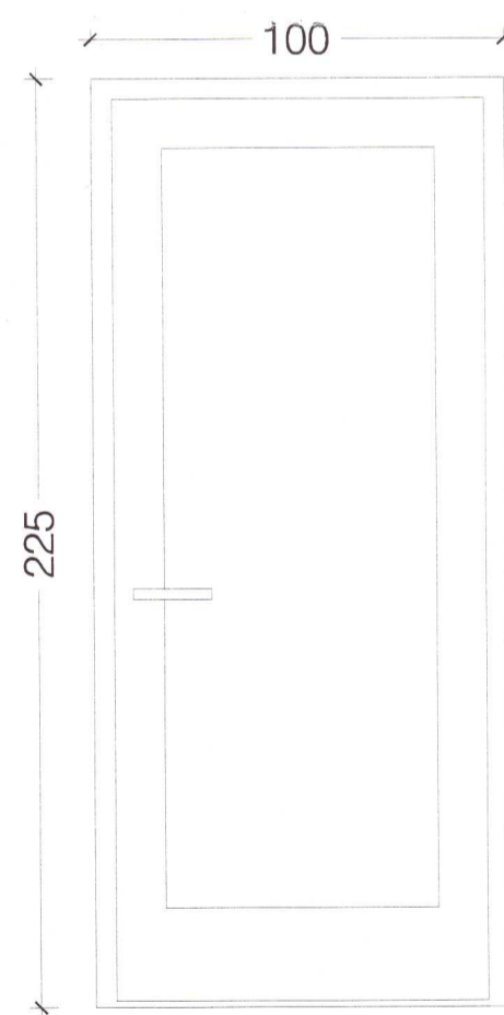
H2 þröskuldur max. 25 mm. Öryggisgler í öllum glerjum. 1 stk.
