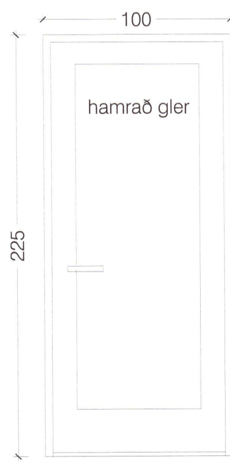
H3 þröskuldur max. 25 mm (útihurð frá snyrtingu ath. m. læsingu) 1 stk.
