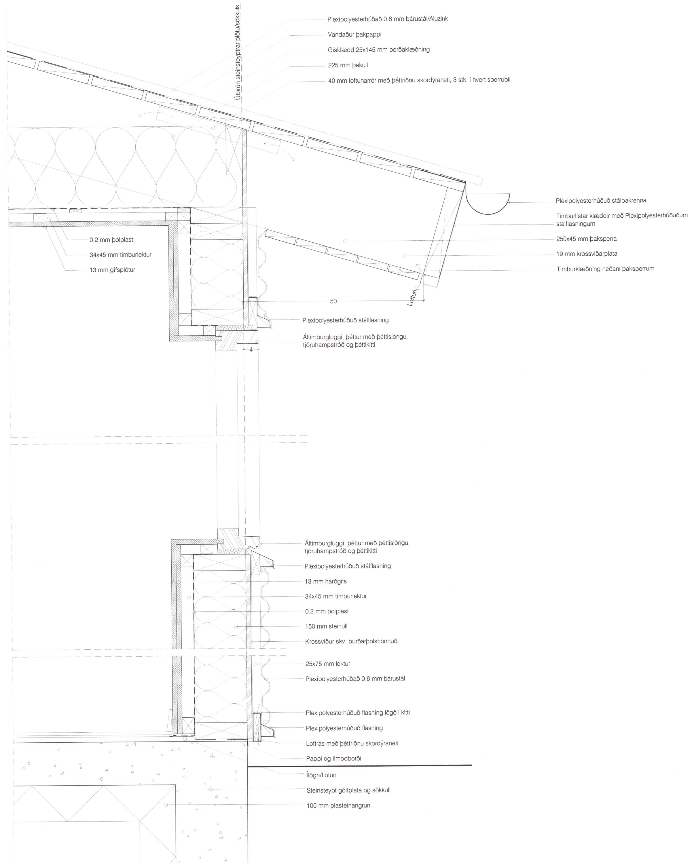
Lóðrétt deili í útvegg og þak í svefnherbergisluta húss - mkv. 1:5
