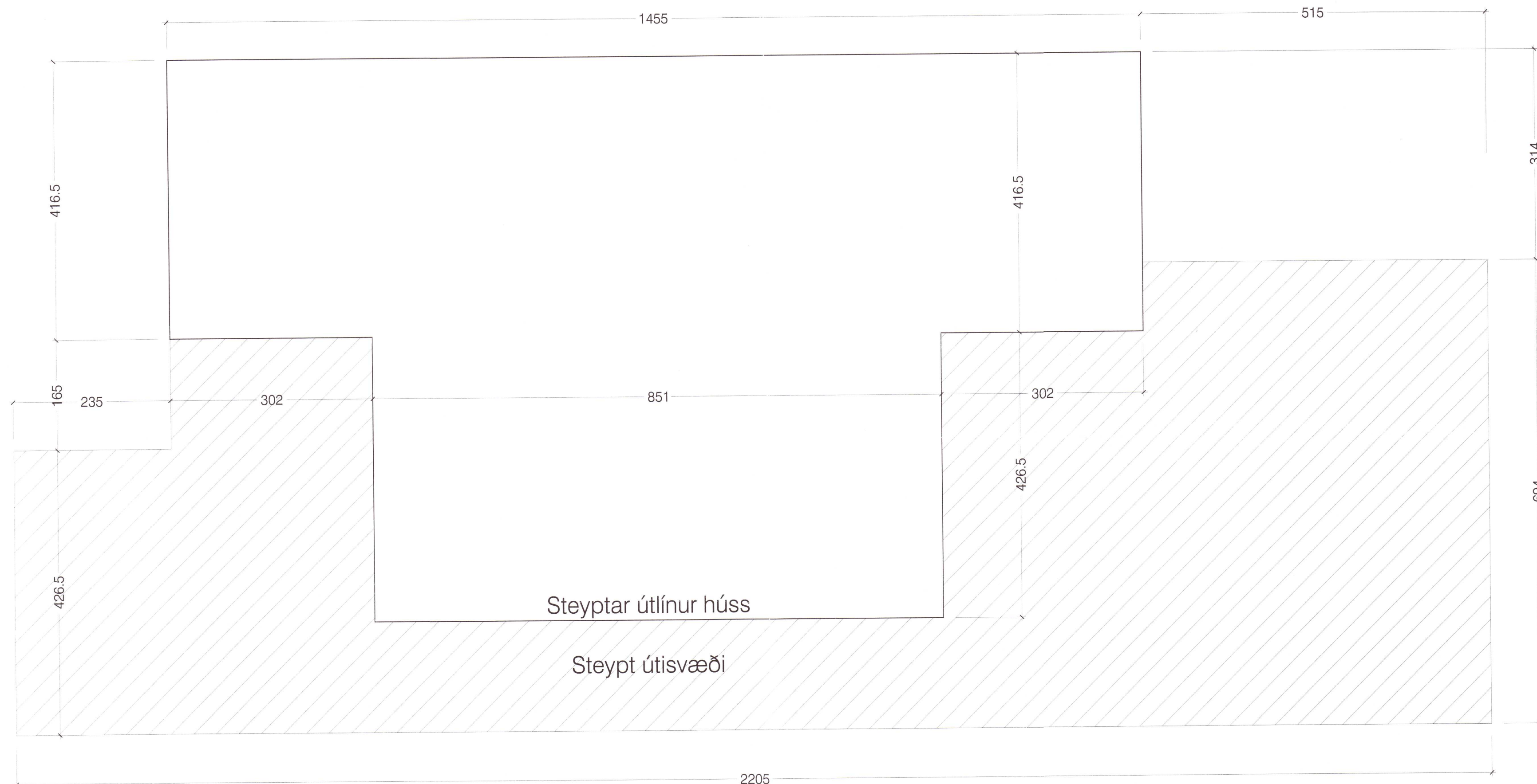
Grunnmynd - mkv. 1:50
