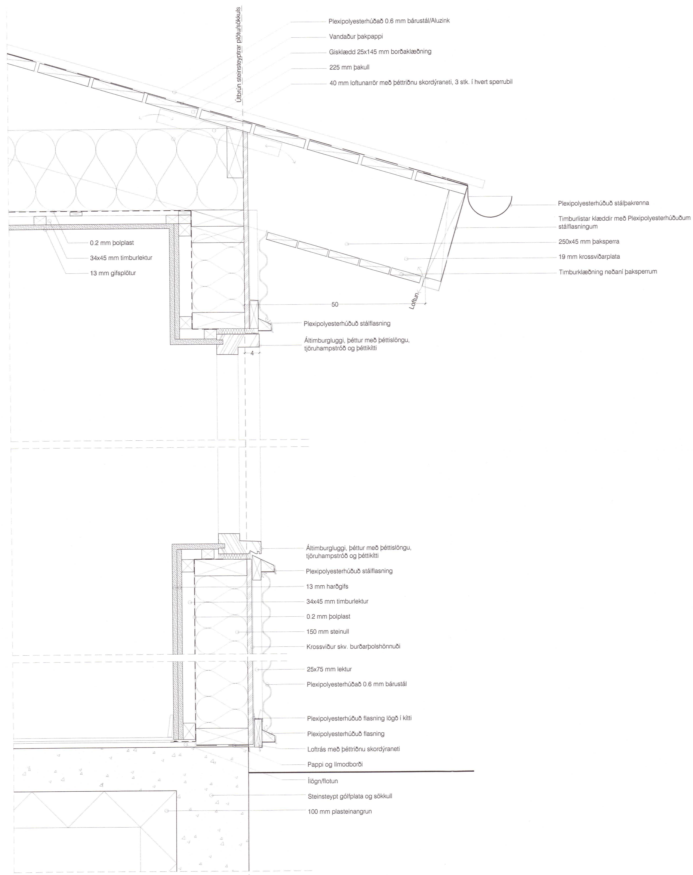
Lóðrétt deili í útvegg og þak í svefnherbergisluta húss - mkv. 1:5
