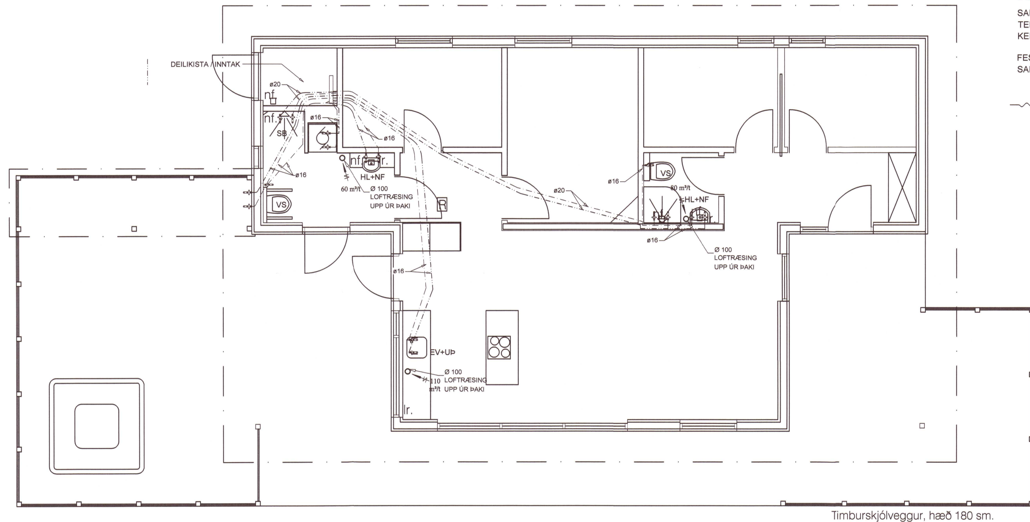
GRUNNMYND NEYSLUVATNSLAGNA, 1:50
