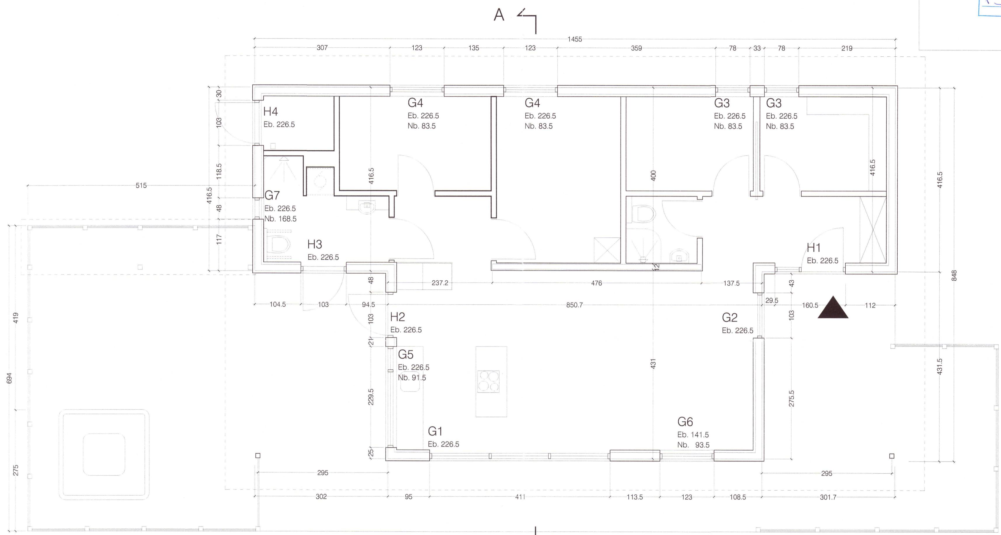
Grunnmynd - mkv. 1:50
