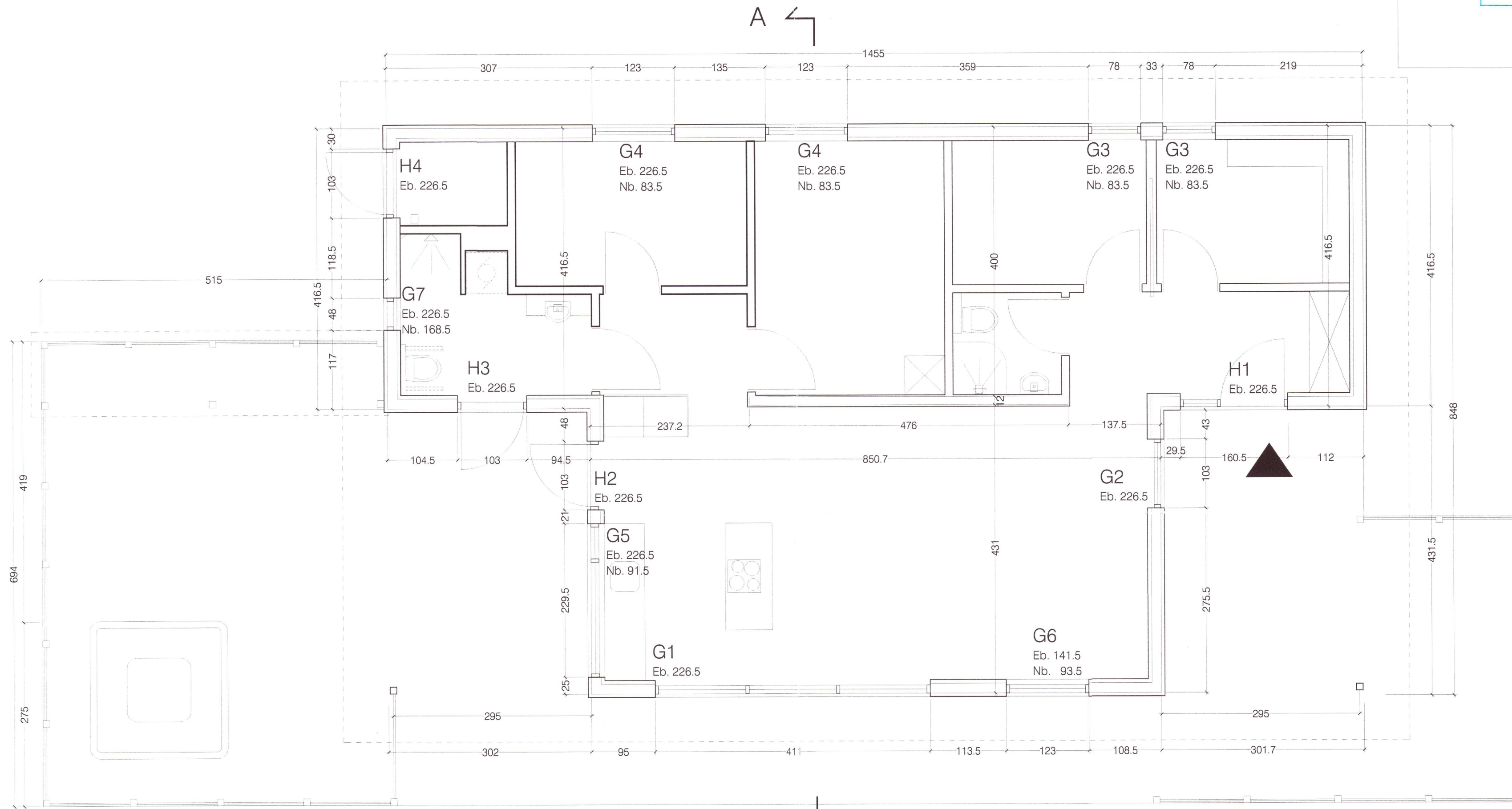
Grunnmynd - mkv. 1:50
