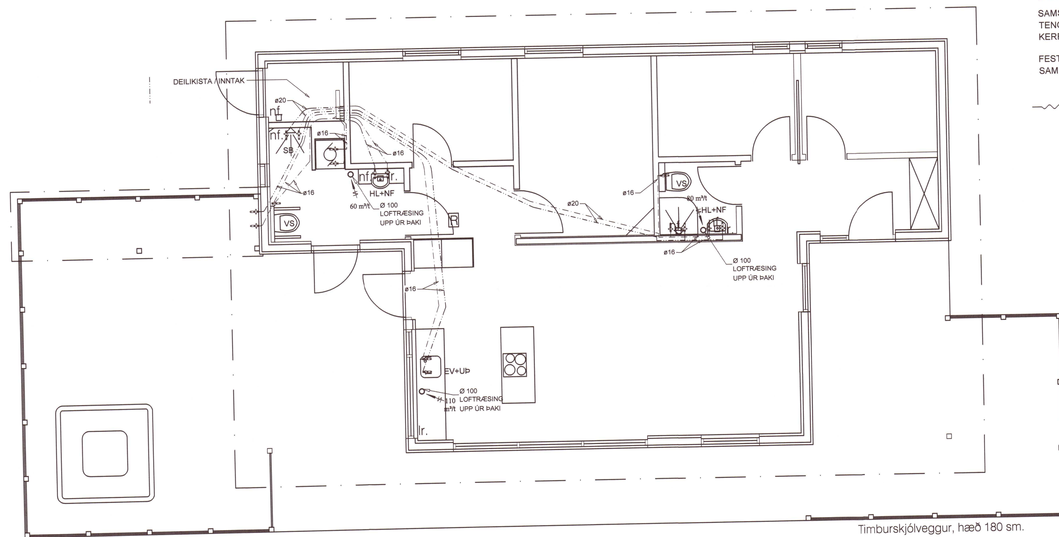
GRUNNMYND NEYSLUVATNSLAGNA, 1:50
