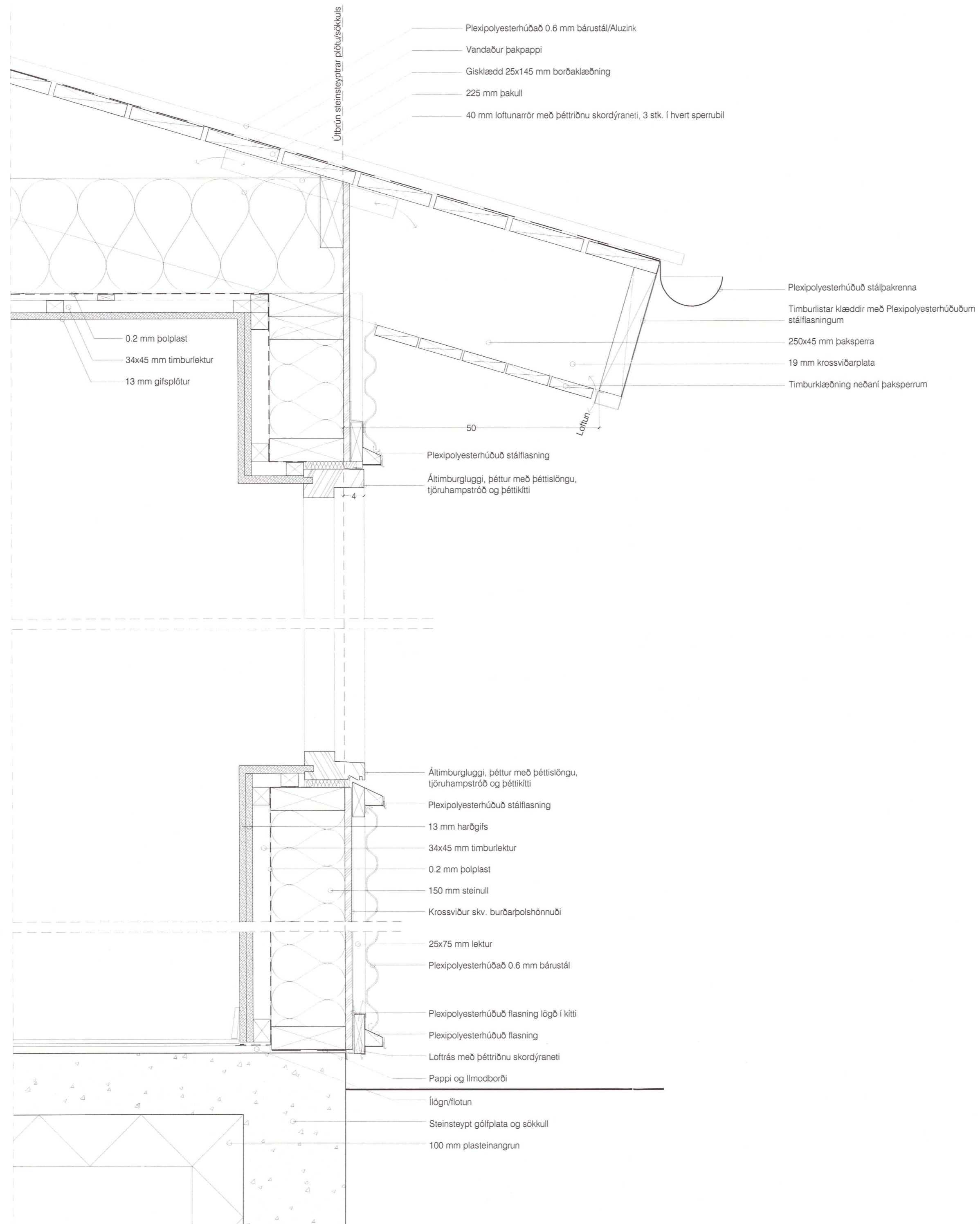
Löðrétt deili í útvegg og þak í svefnherbergisluta húss - mkv. 1:5
