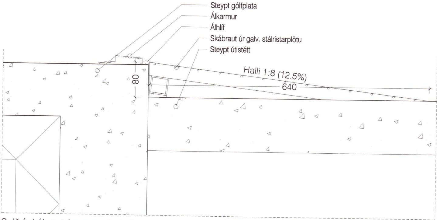
Snið í skábraut framan við aðalinngang og svalahurð - mkv. 1:5
