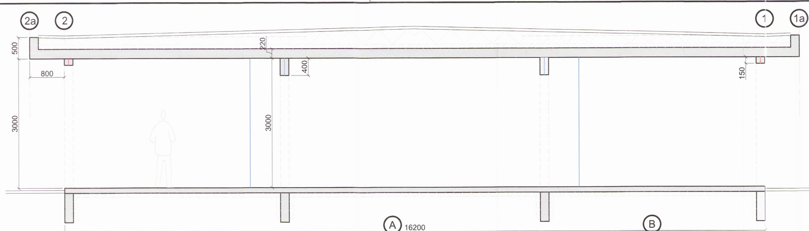
Snið A Mkv. 1:50
