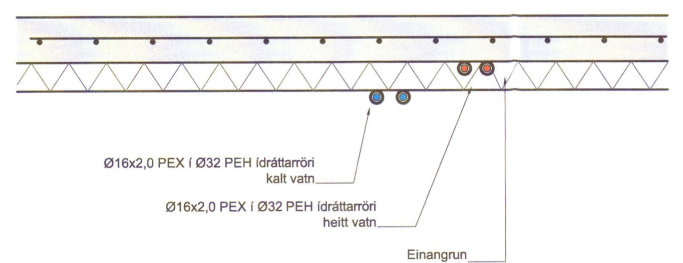
Staðsetning neysluvatnslagna í gólfi M 1:10
