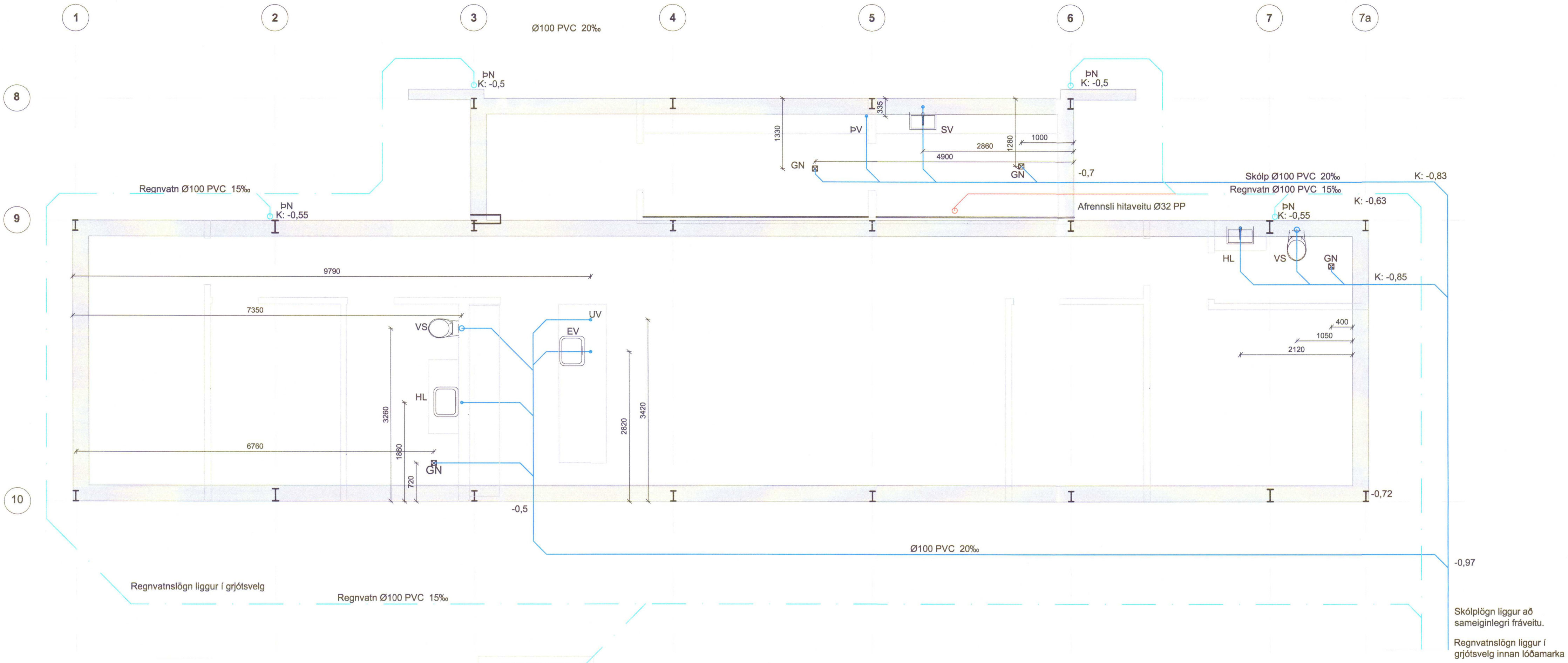
Grunnmynd frárennislagna M 1:50
