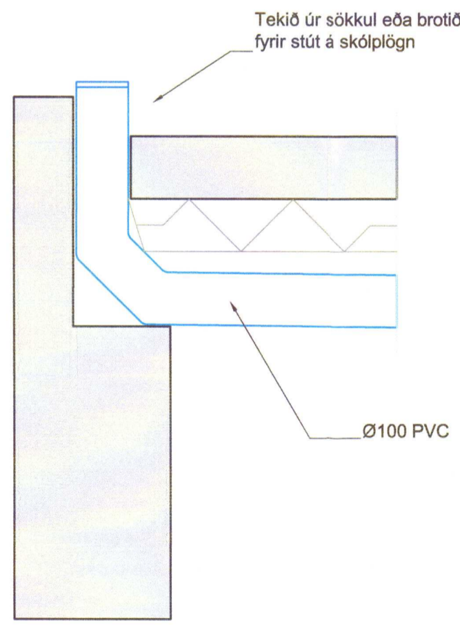
Snið í skólplögn M 1:10
