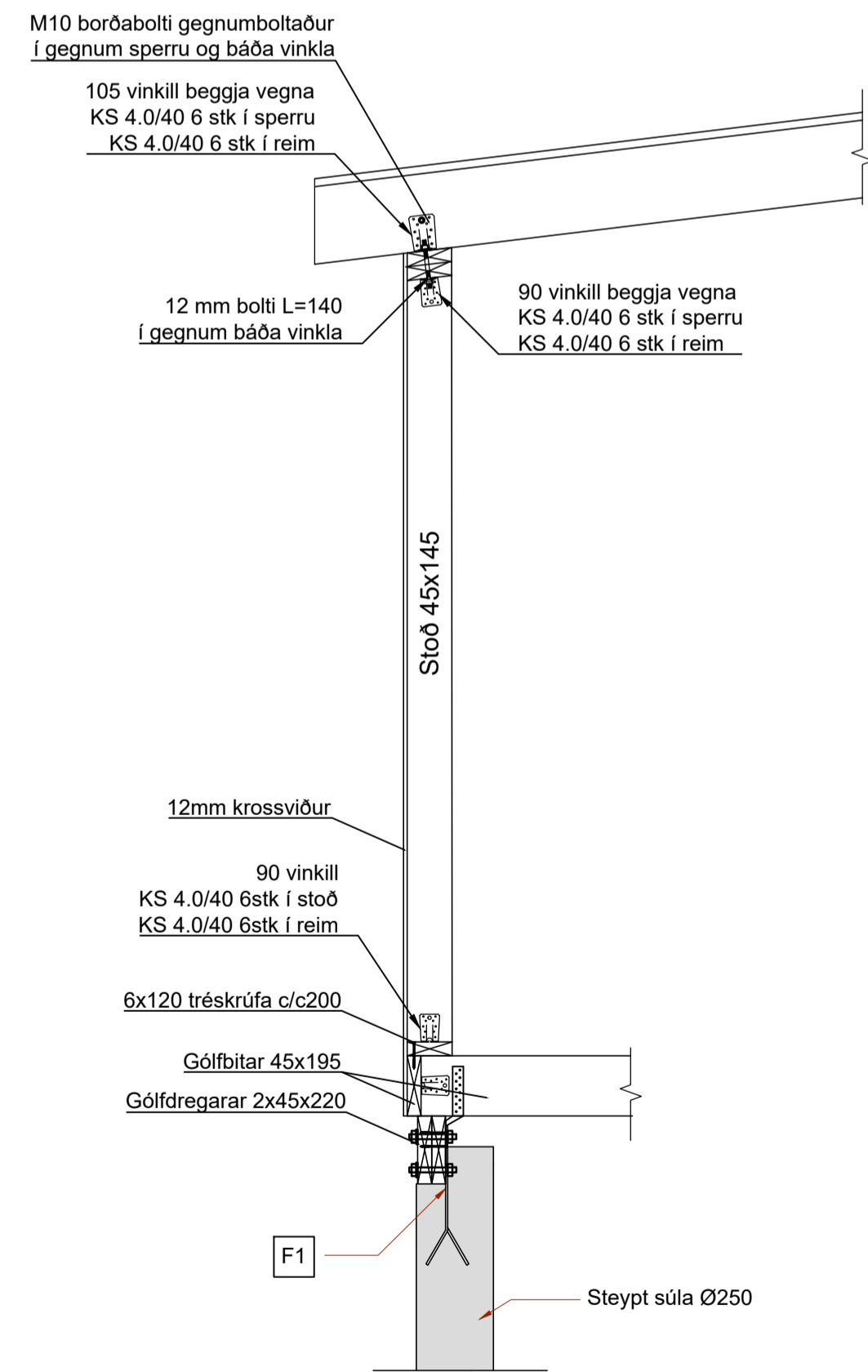
SNID B1 MKV. 1:20
