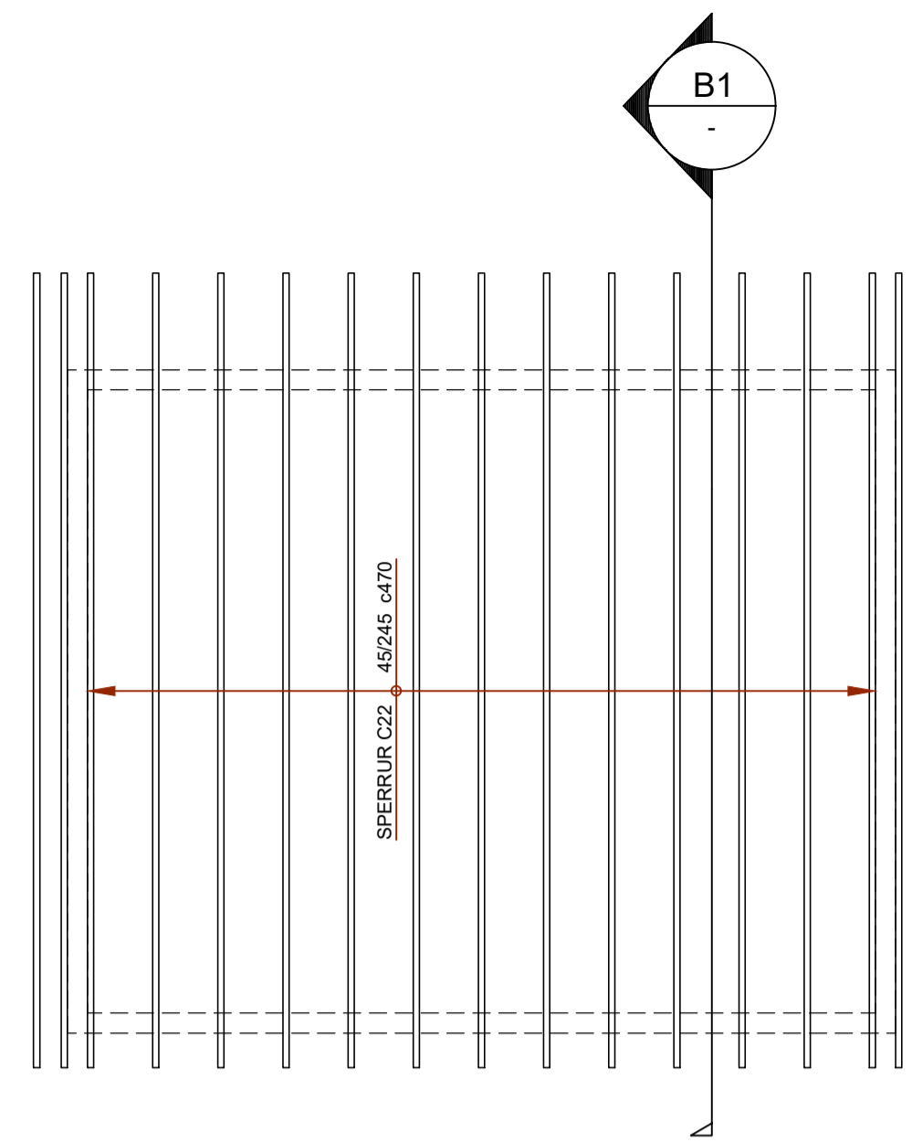
GRUNNMYND ÞAKVIRKI MKV. 1:50
