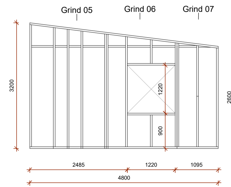
ÁSYND VEGGJAGRINDA MKV. 1:50
