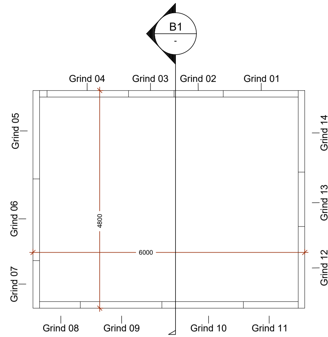
GRUNNMYND VEGGIR MKV. 1:50
