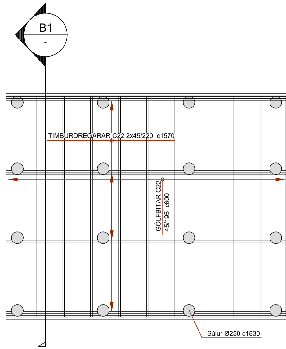
GRUNNMYND UNDIRSTÖÐUR - GÓLFBITAR MKV. 1:50
