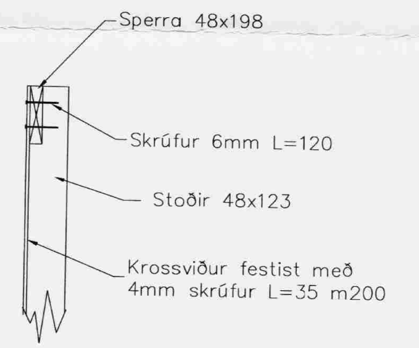
B Snið 1 = 20 mm
