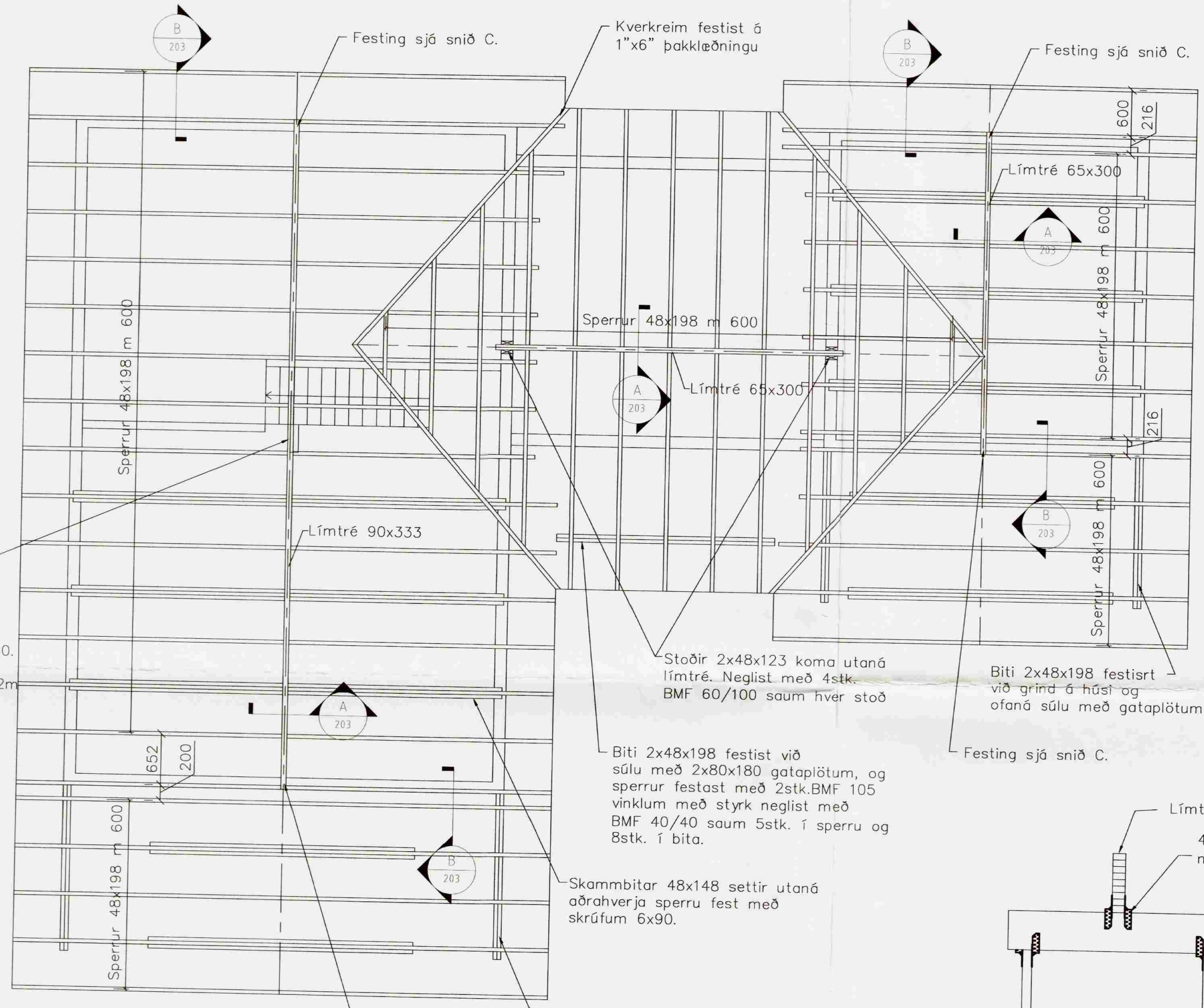
Grunnmynd þaks 1 = 50 mm
