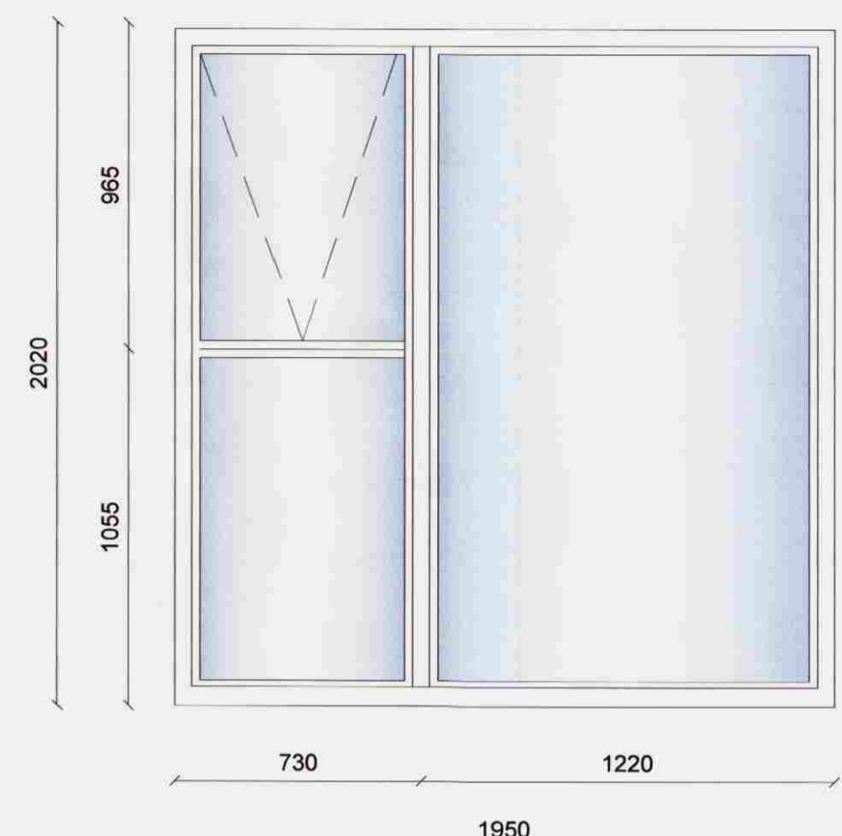
G-10 Opnun .....Topphengd Fjöldi ..... 1.stk.
