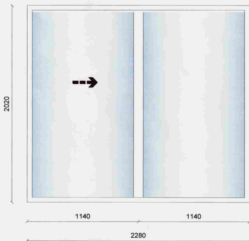
G-8 Opnun loftunar.....Frá vinstri til hægri Fjöldi ..... 1.stk.
