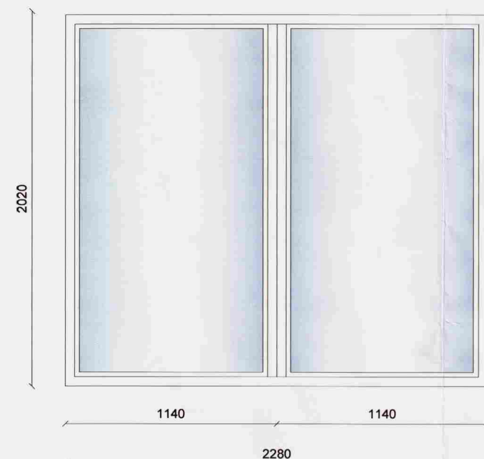
G-9 Fjöldi ..... 1.stk.
