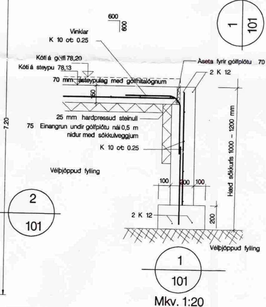
Mkv. 1:20
