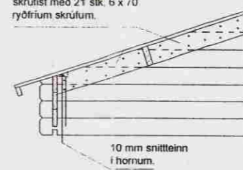
STYRKING Í GAFLI 1 : 20
