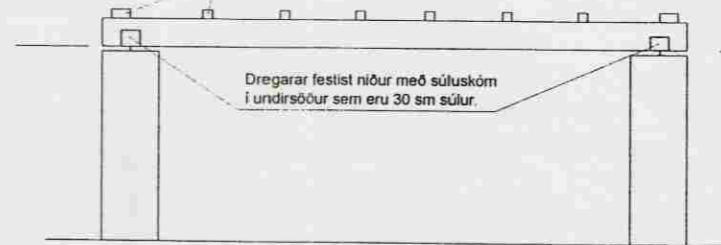
SNID A - A 1 : 20
