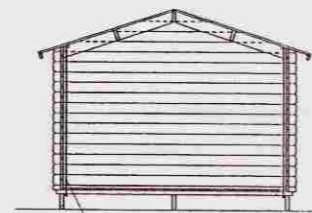
SNID Í HÚSI 1 : 50
